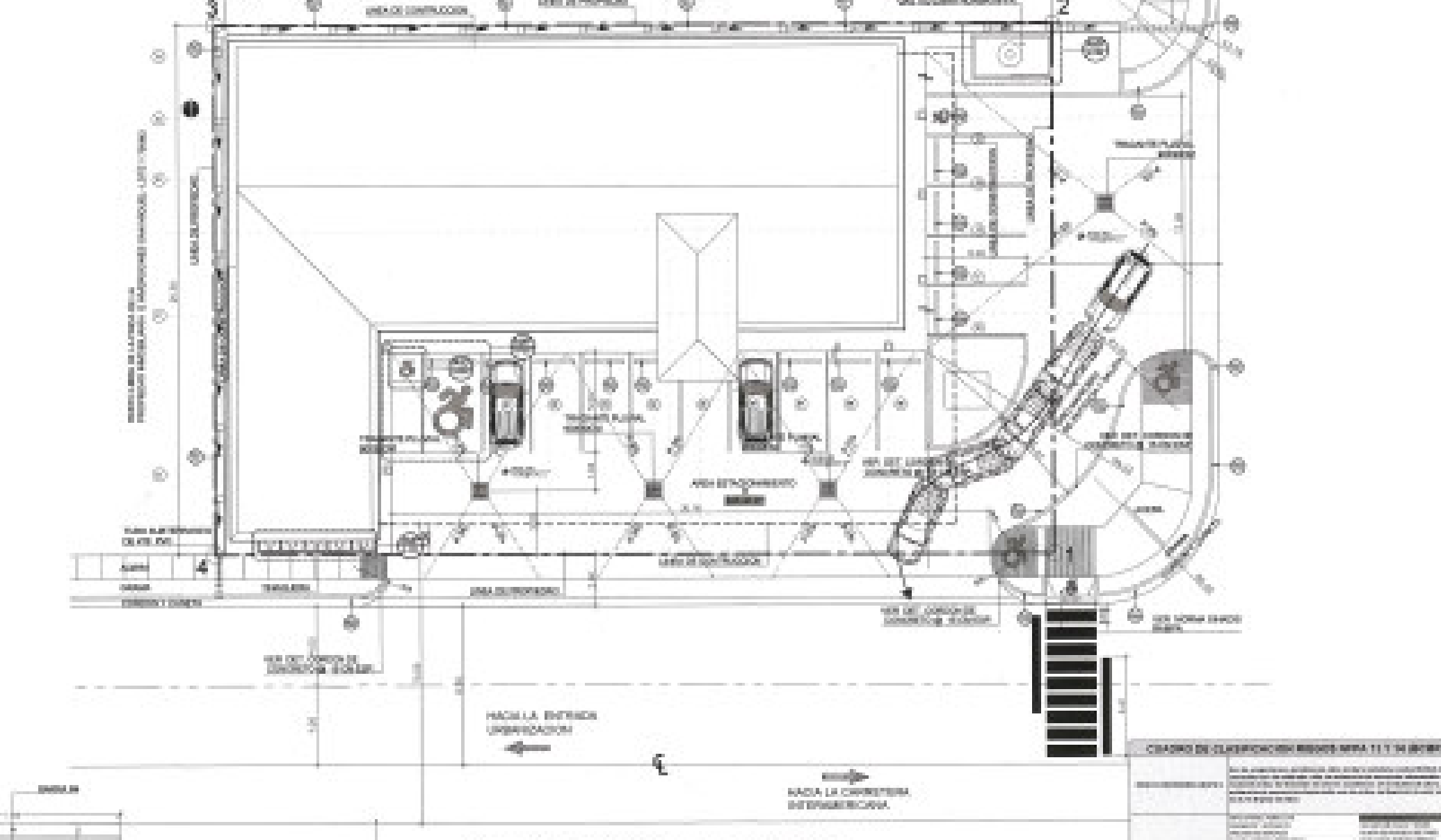
LOCALIZACION GENERAL ESC. 1:150
