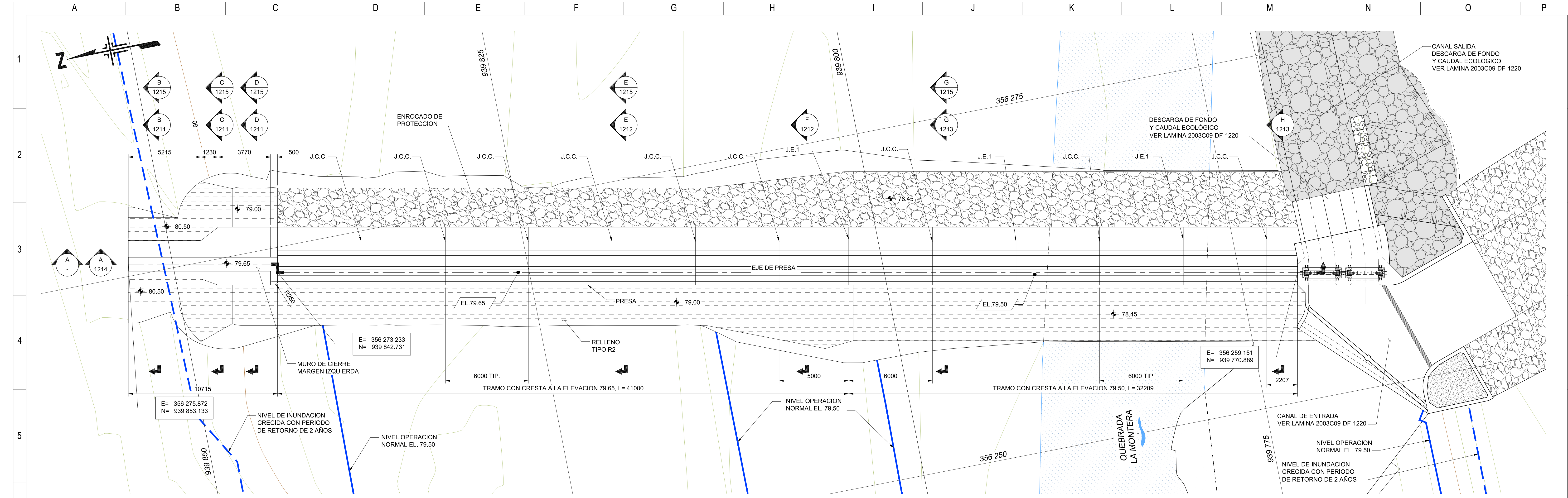
PLANTA ESCALA 1:125
