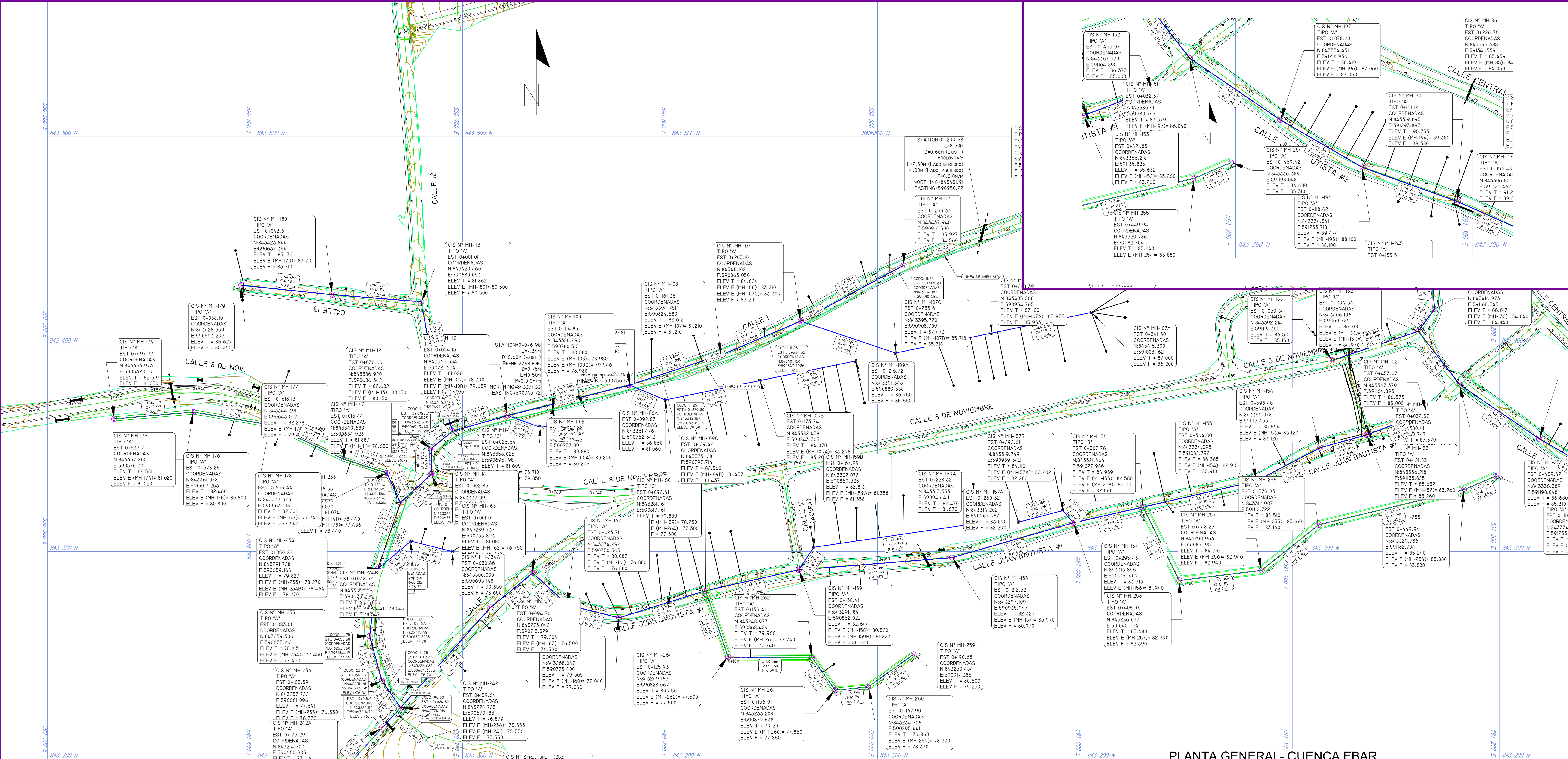
PLANTA GENERAL- CUENCA EBAR
