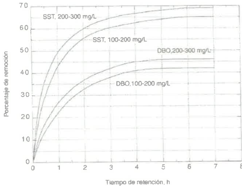
Figura 67. Valores usuales para la remoción de sólidos y DBO en un tanque de sedimentación primaria Tomado de Crites y Tchobanoglous, 2000, p.304
