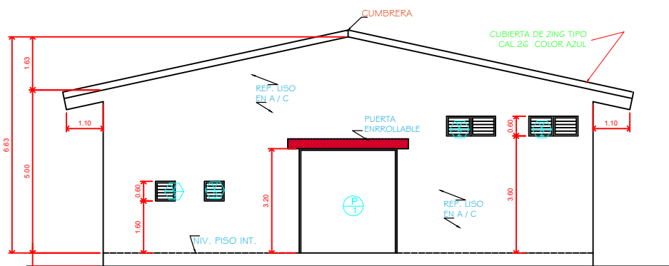
VISTA LATERAL IZQUIERDO ESC: 1:75
