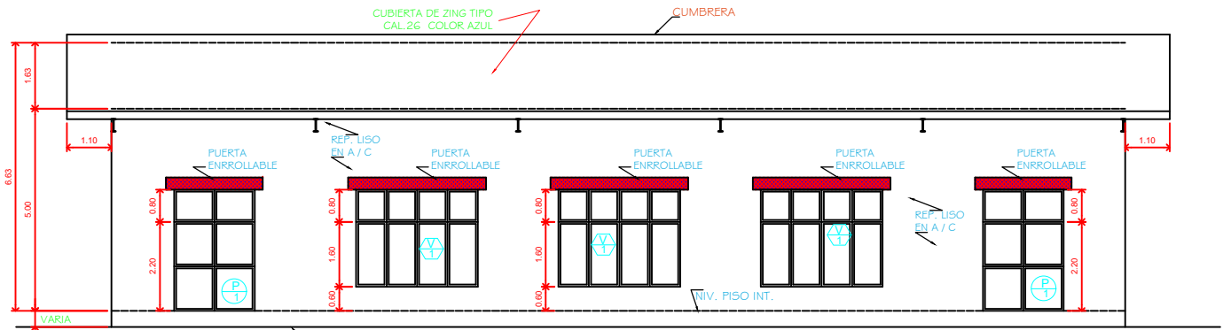
ELEVACION PRINCIPAL ESC: 1:75
