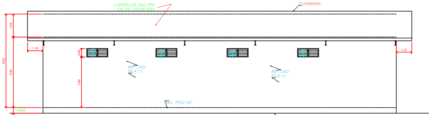
ELEVACION POSTERIOR ESC: 1:75
