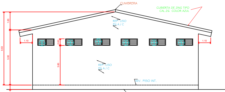
VISTA LATERAL DERECHO ESC: 1:75
