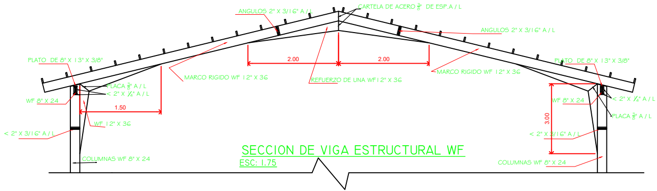
SECCION TRANSVERSAL DE LOCAL ESC: 1:75
