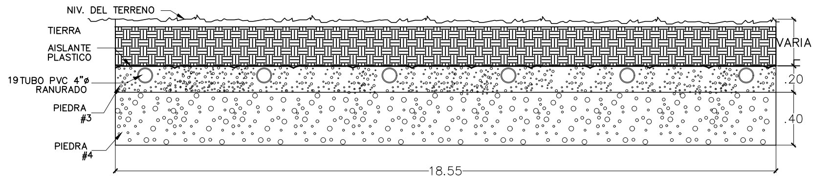
SECCIÓN LECHO DE PERCOLACIÓN ESCALA S/E
