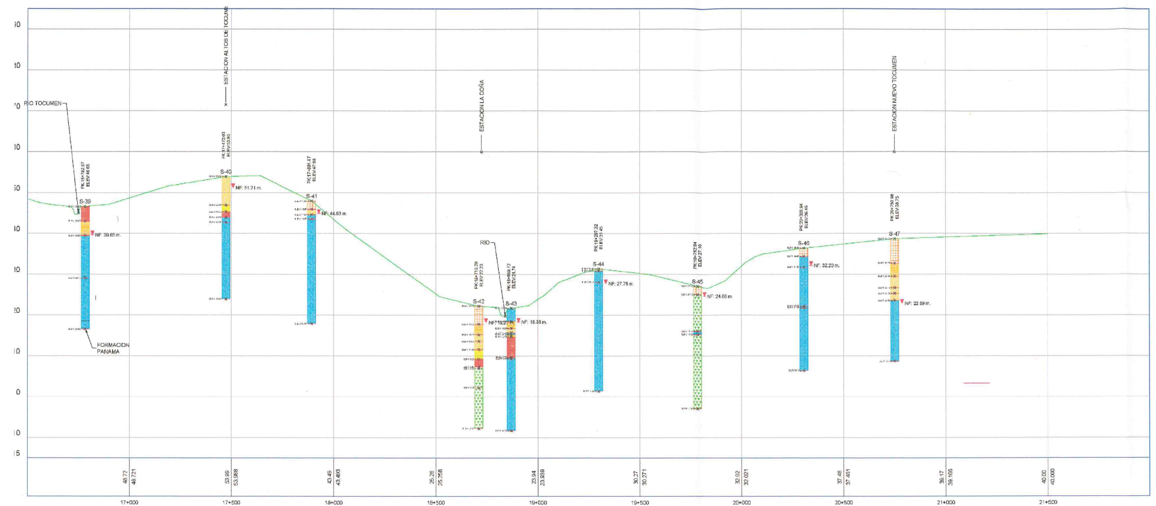
FIGURA N° 4 PERFIL GEOLOGICO (Estación de Altos de Tocumen hacia Estación Nuevo Tocumen)
