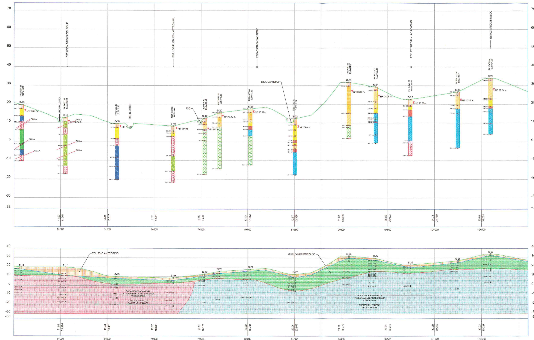
FIGURA N° 2 PERFIL GEOLOGICO (Estación de Brisas del Golf hacia Estación Don Dosco)
