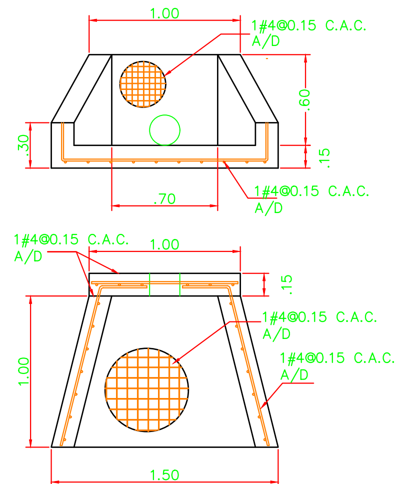
DETALLE ESTRUCTURAL CANAL DE SALIDA PTAR
