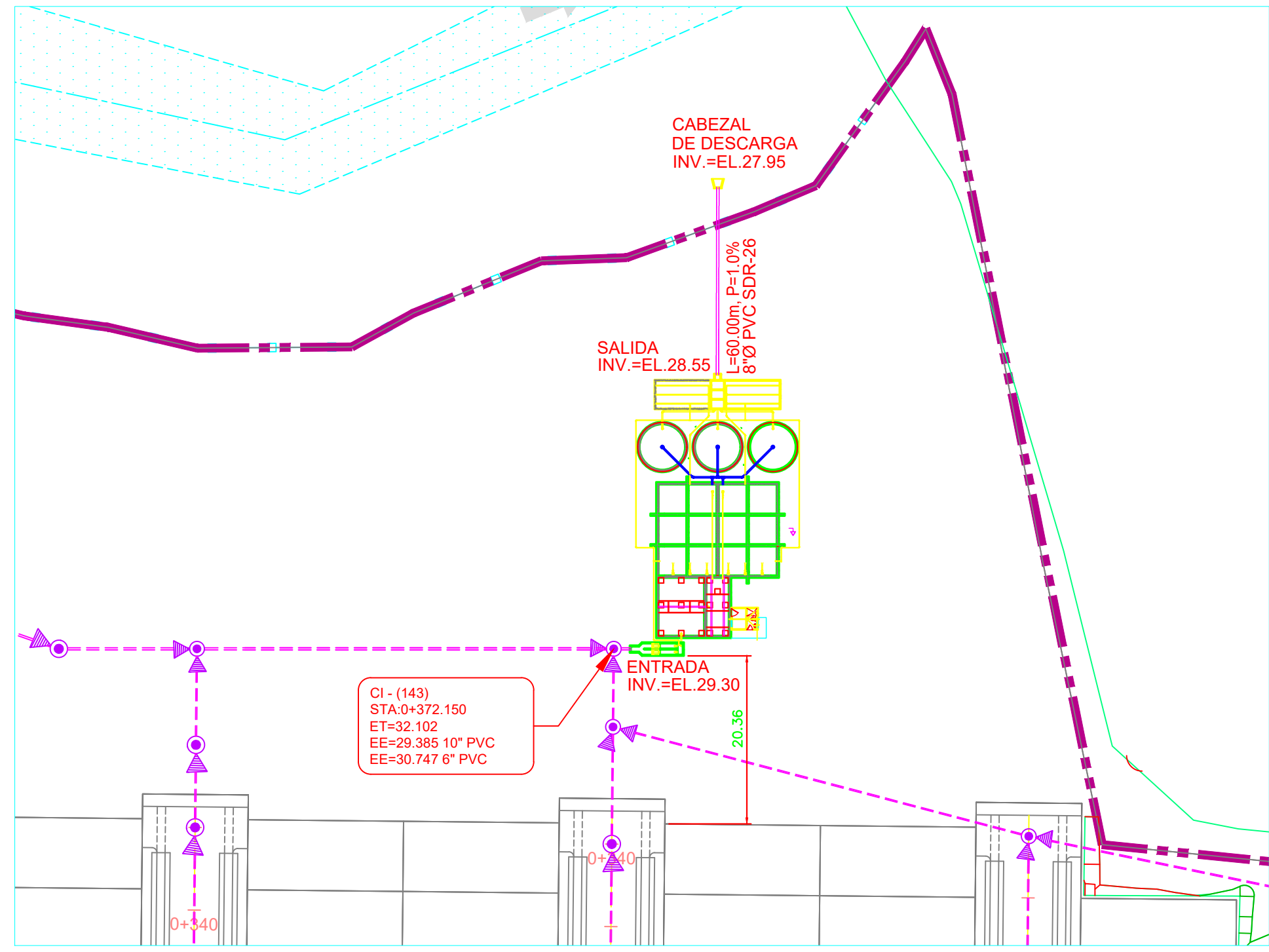
PLANTA DE UBICACIÓN DE PTAR ESC: 1: 500
