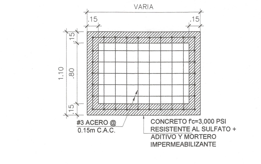
DETALLE CONSTRUCTIVO TIPOICO DE CAJA DE CONCRETO
