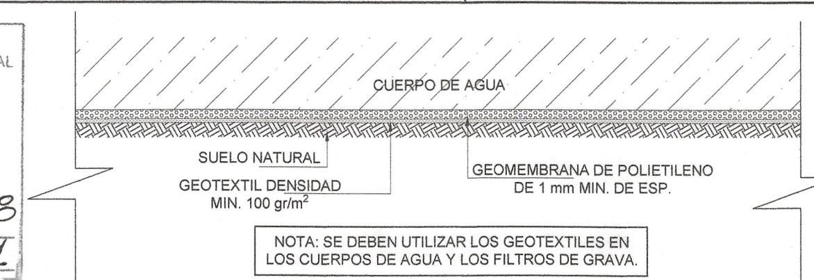
DETALLE IMPERMEABILIZACION DE LAGUNAS Y FILTROS DE GRAVA
