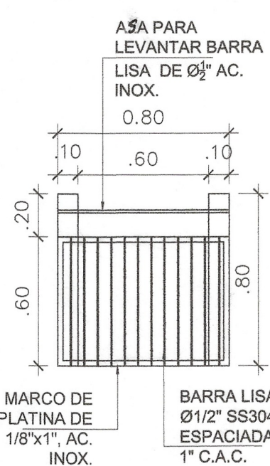
DETALLE DE REJILLA TIPO 2
