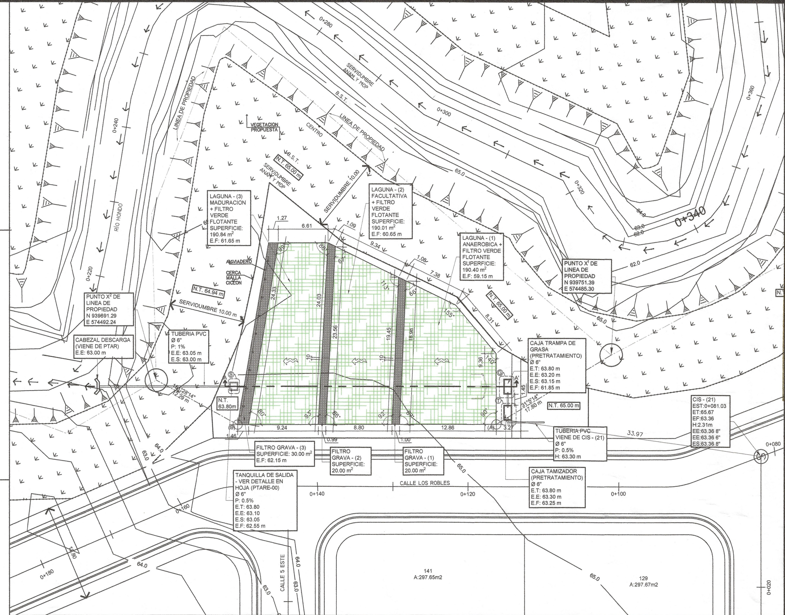
PTARE - PLANTA DE TRATAMIENTO
