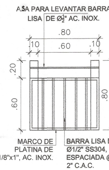
DETALLE DE REJILLA TIPO 1
