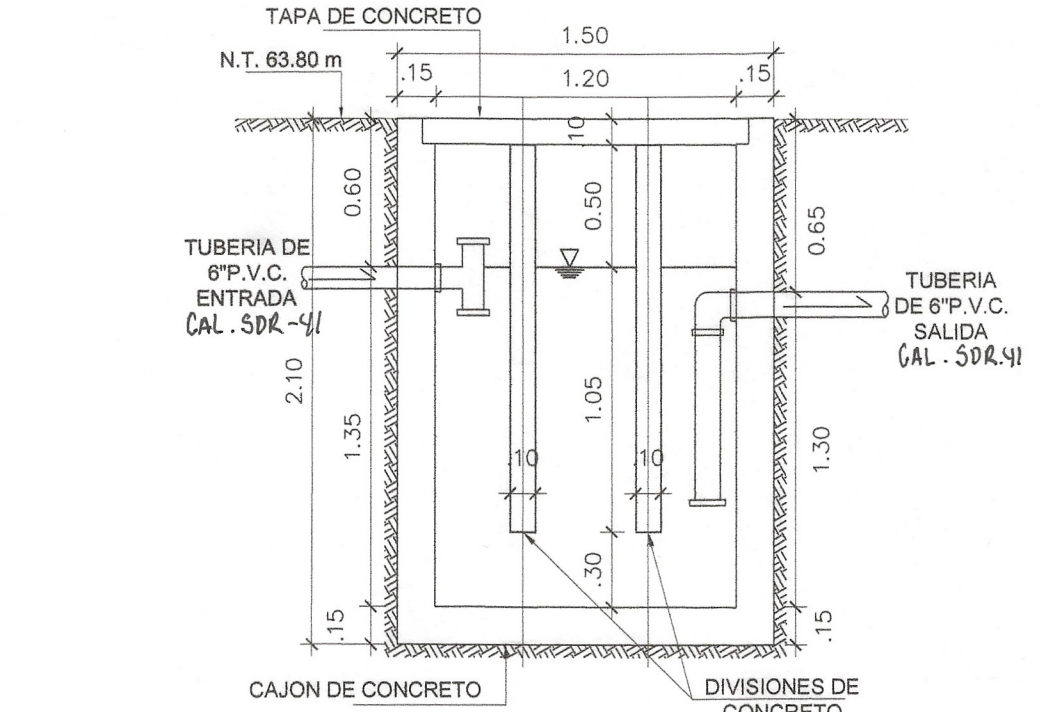
SECCION S-S' - CAJA TRAMPA DE GRASA (PRETRATAMIENTO)
