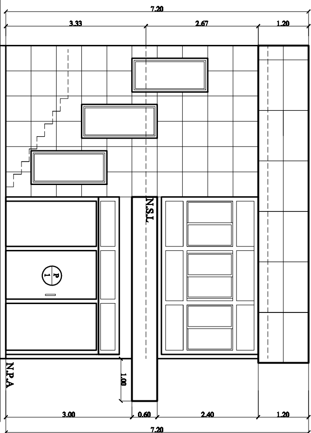
FACHADA FRONTAL. ESC: 1:50
