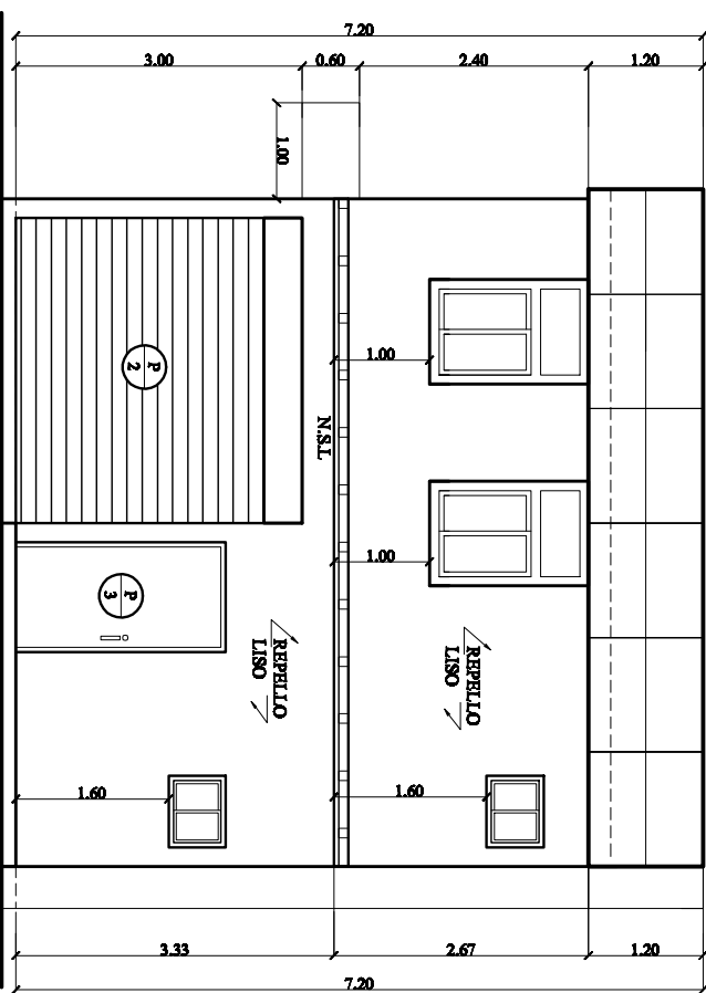
FACHADA POSTERIOR. ESC: 1:50
