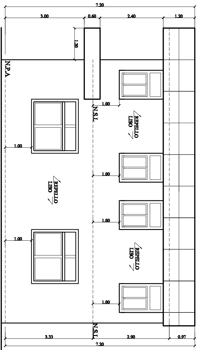
FACHADA LATERAL DERECHA. ESC: 1:50
