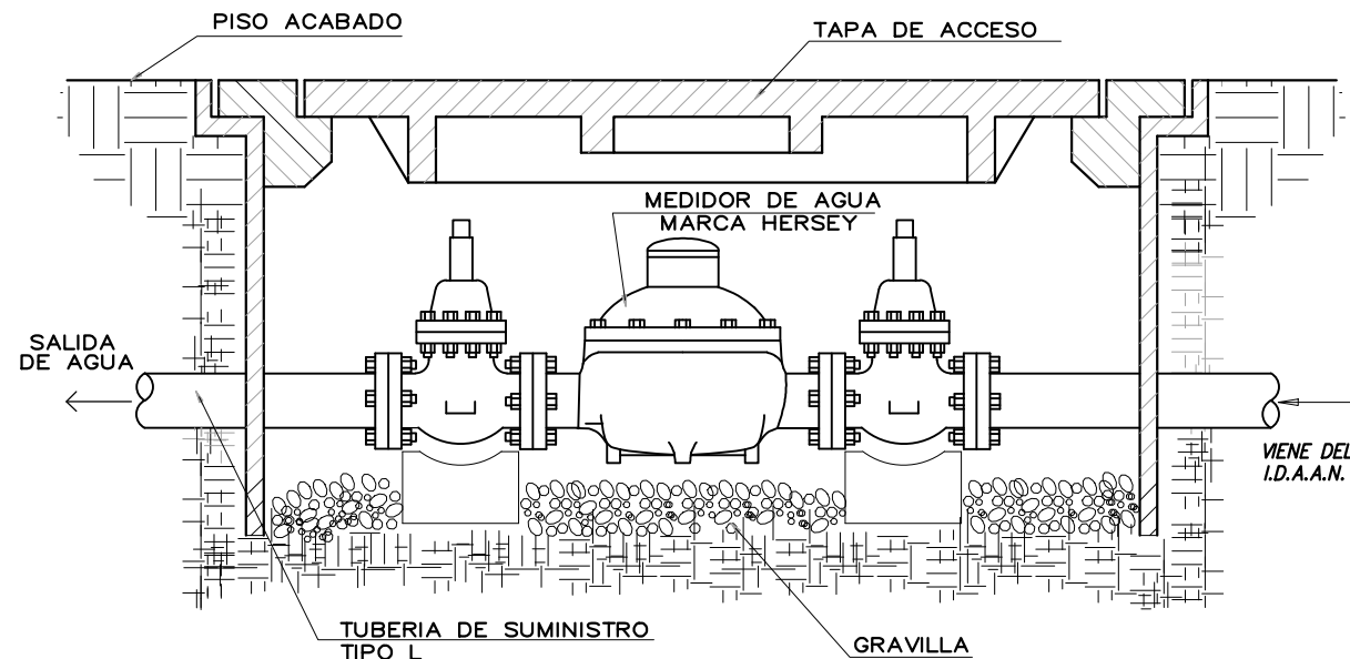
DETALLE DE INSTALACION MEDIDOR MAESTRO NIVEL -100 SIN ESCALA
