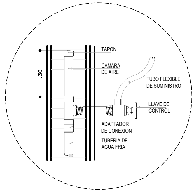
DET. LLAVE DE PASO PARA SUMINISTRO DE AGUA EN ARTEFACTO SANITARIO SIN ESCALA
