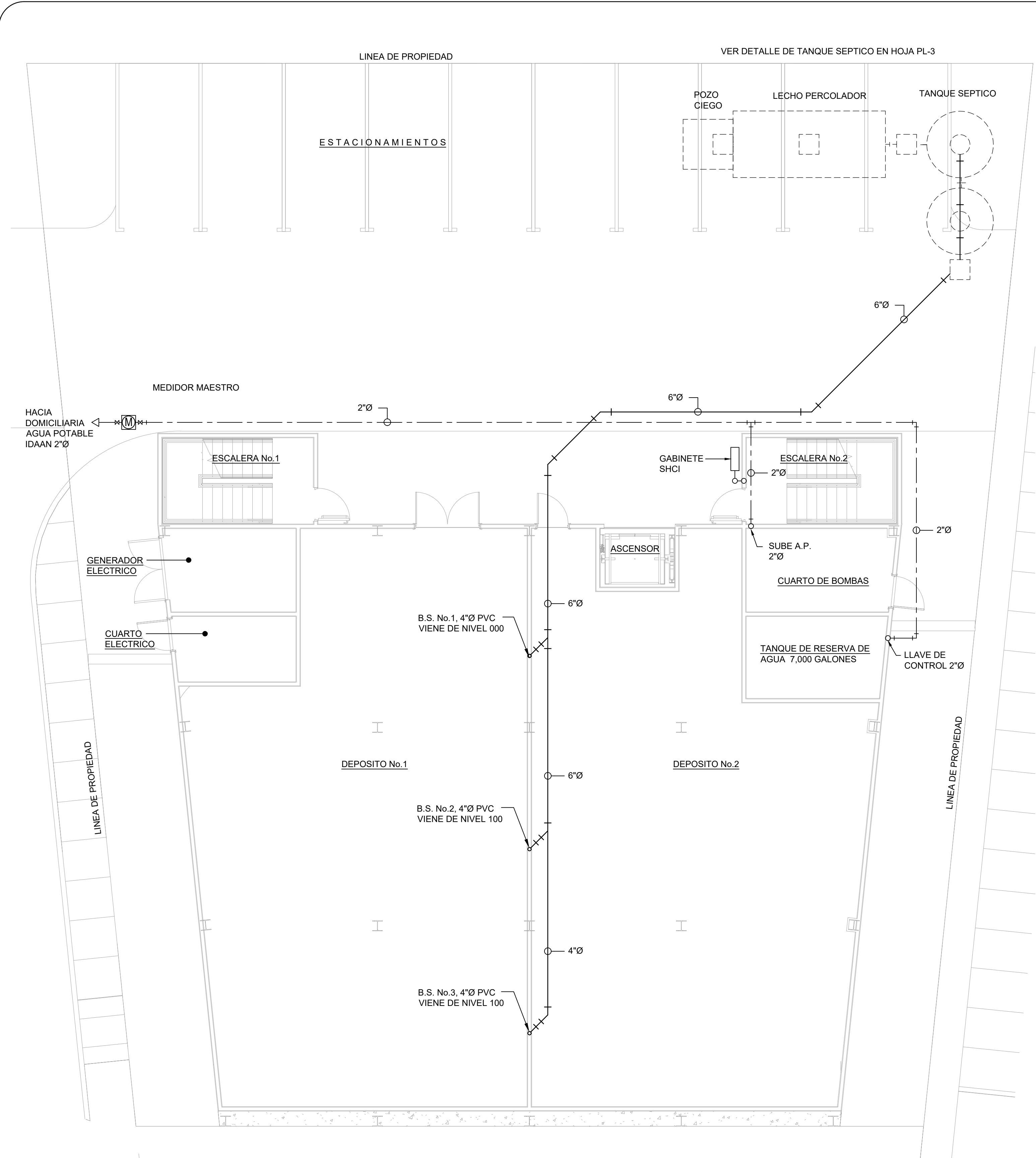
PLANTA DE PLOMERIA NIVEL -100 ESCALA 1:75
