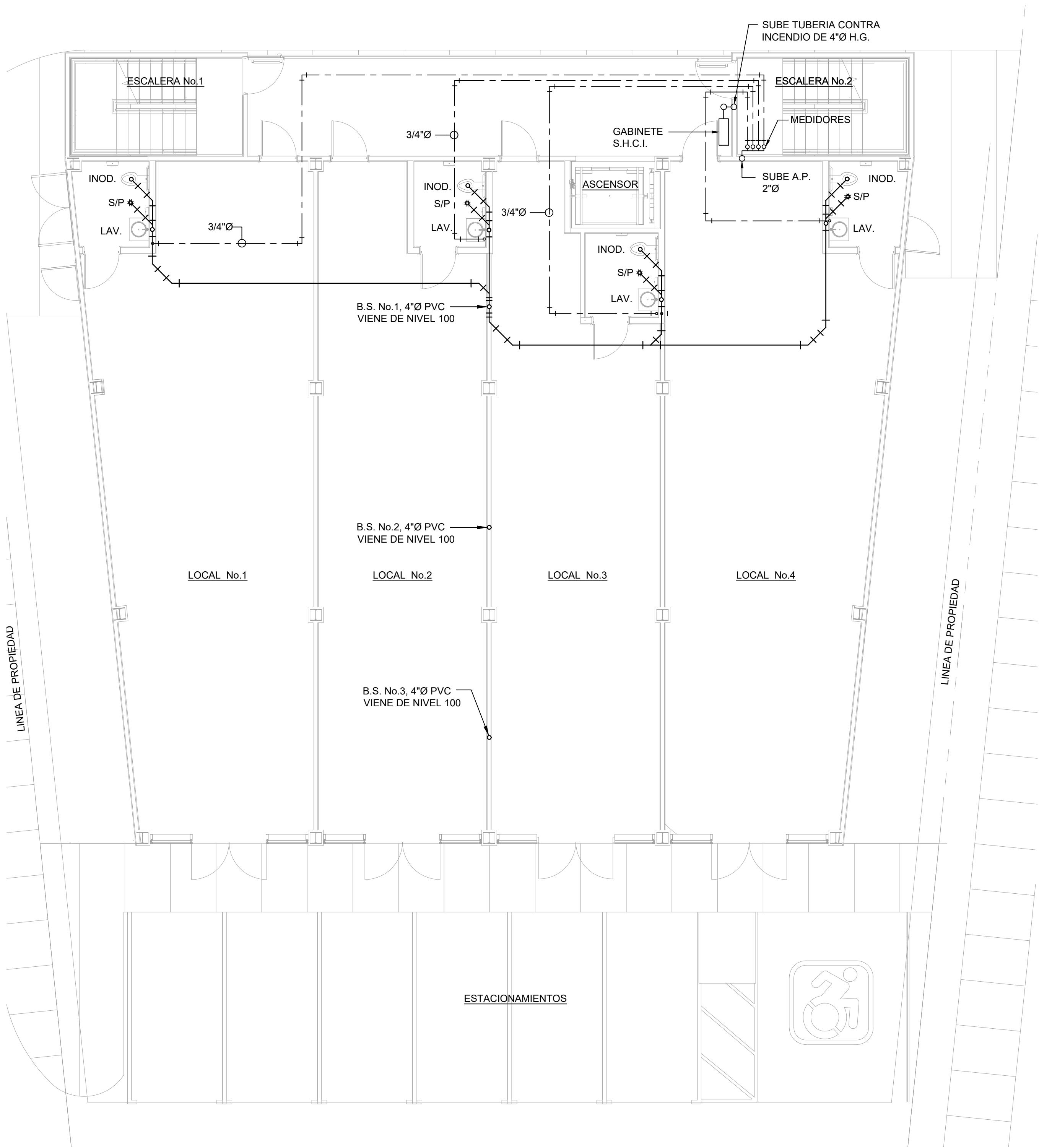
PLANTA DE PLOMERIA NIVEL 000 ESCALA 1:75
