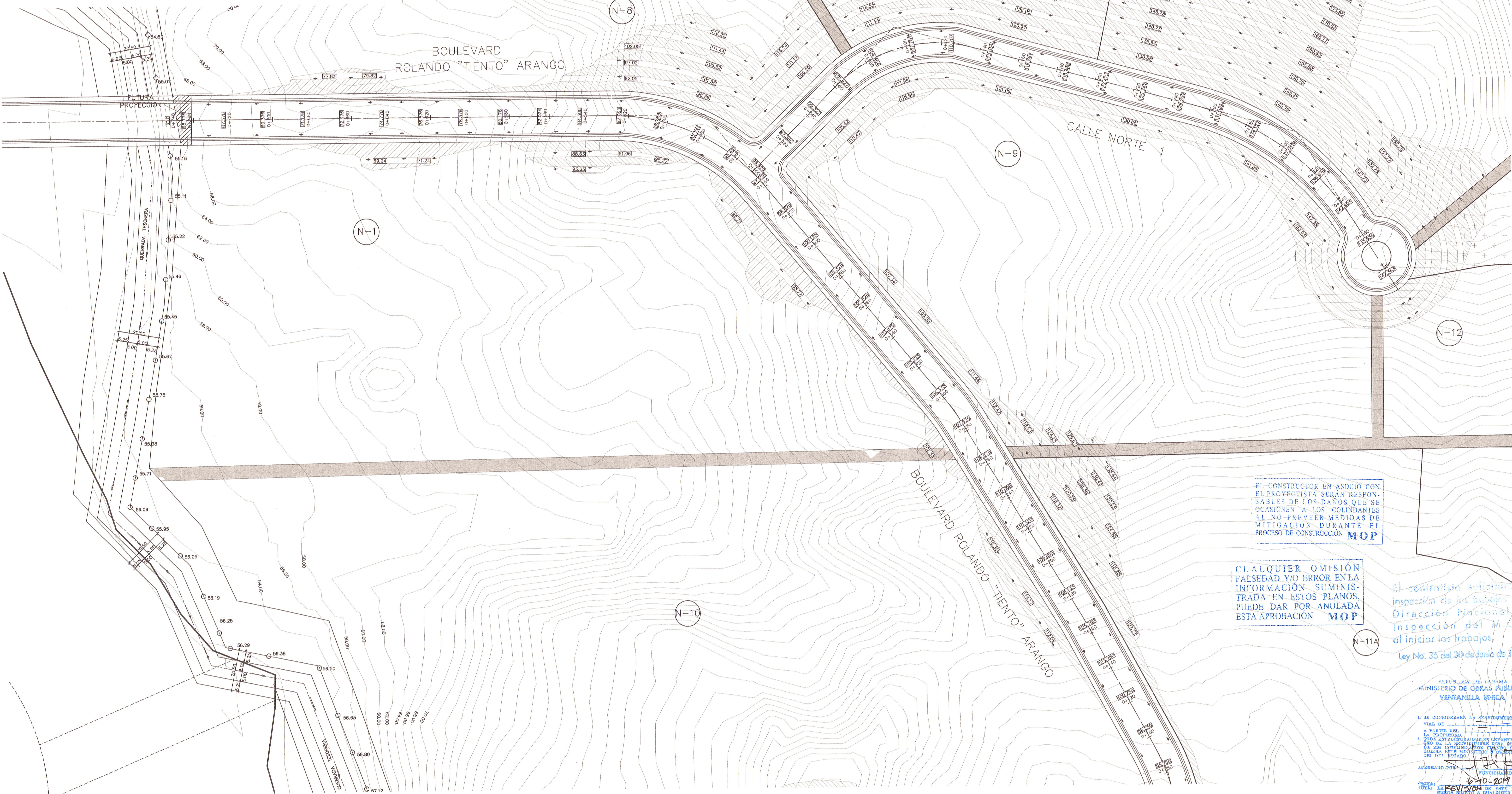
PLANTA DE TERRACERIA - AREA NORTE (SECTOR-N1) ESCALA = 1 : 750
