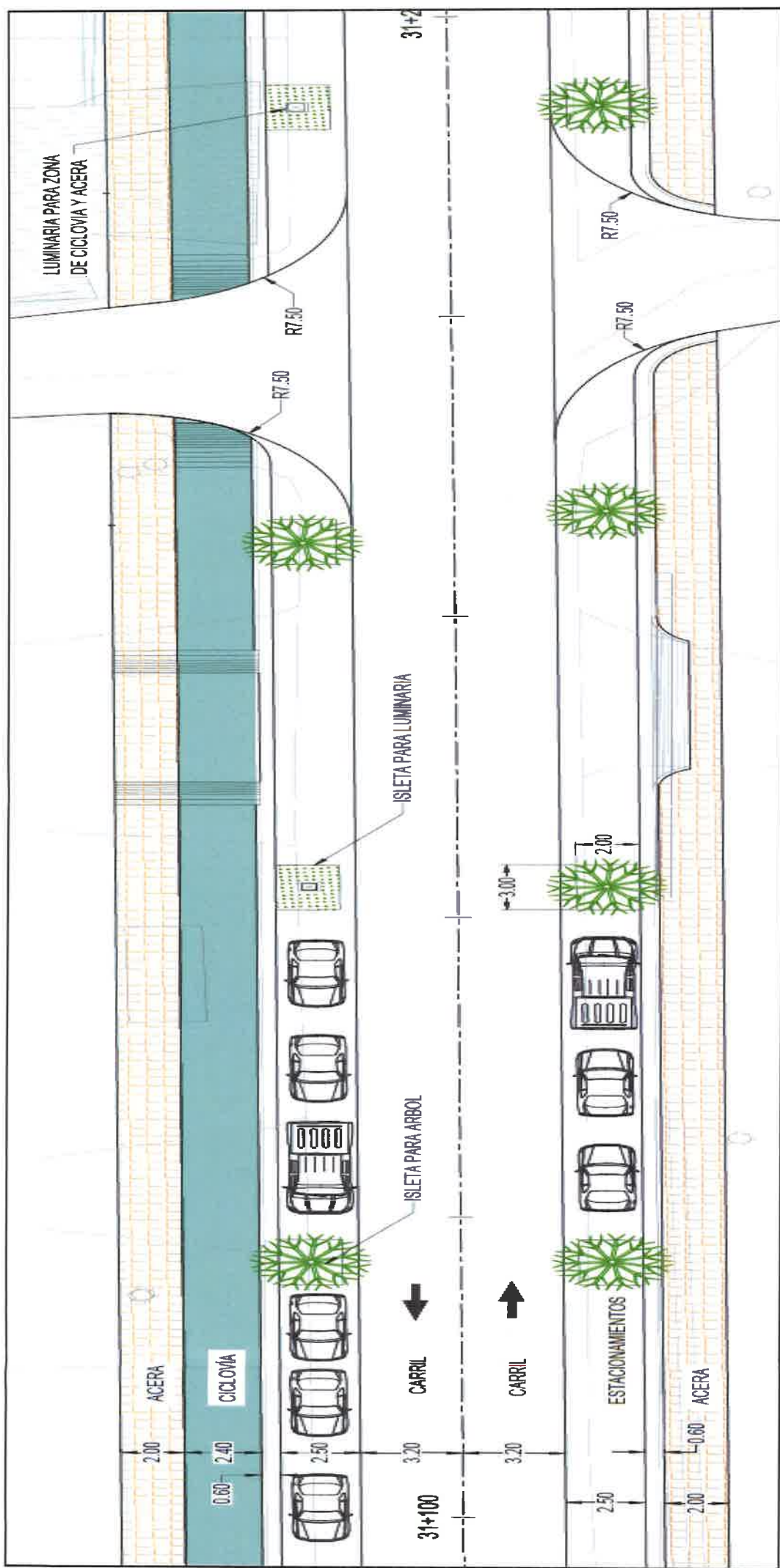
Plano 4: Planta Demostrativa (Volcán), sometida en esta Solicitud de modificación del EsIA cat II Estudio, Diseño y Construcción para la Rehabilitación y ensanche de la carretera Concepción (cpa)- Cuesta de Piedra – Volcán”
