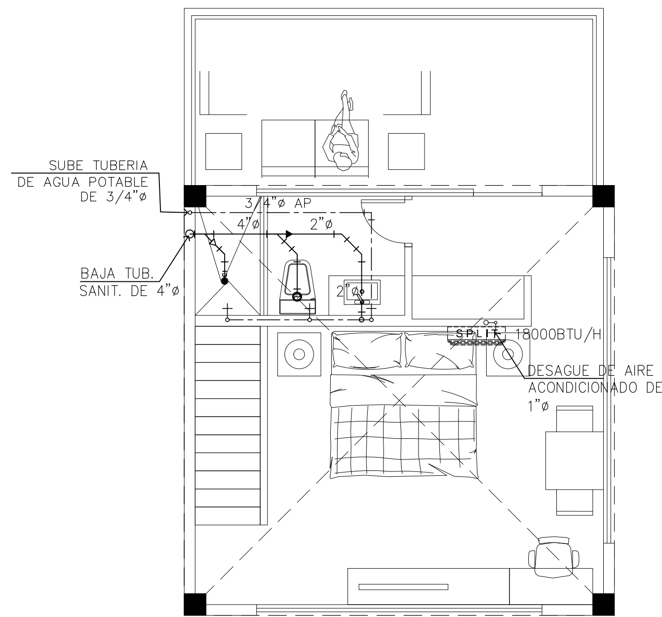
HABITACION #1 P.A. A= 49 M2
