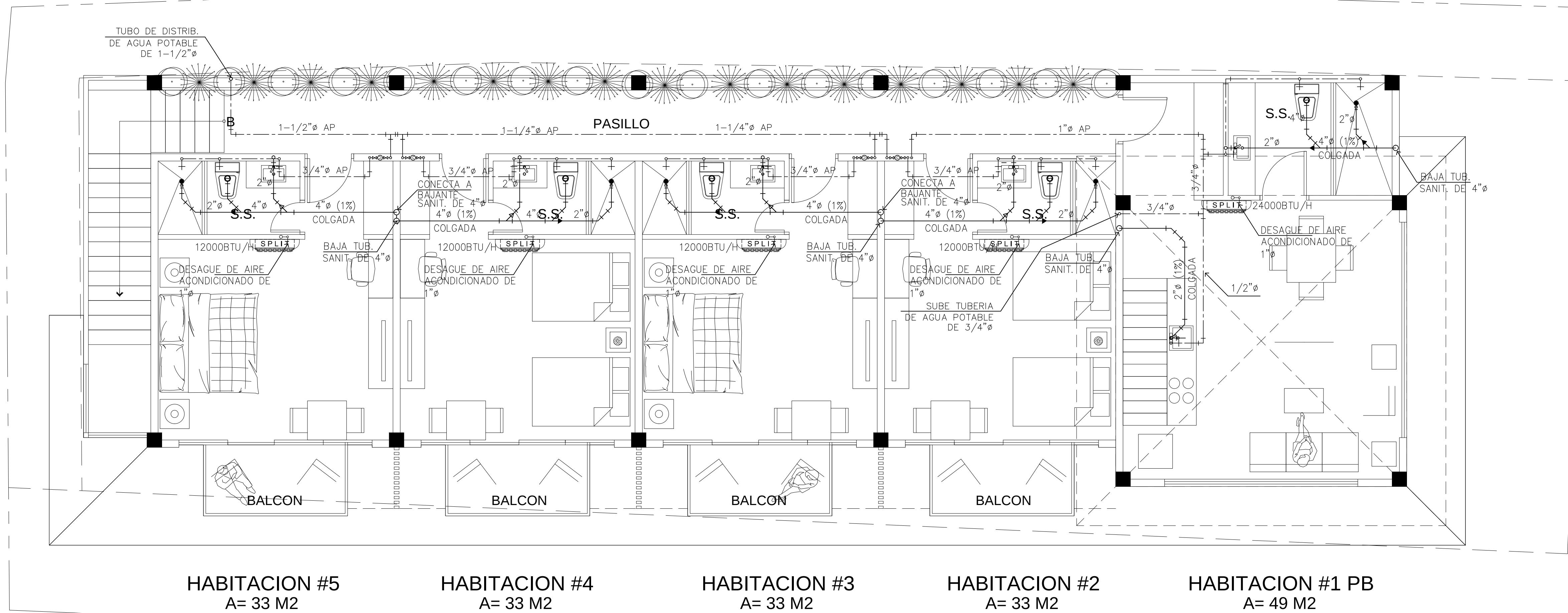
PLANTA DE DISTRIBUCION DE PLOMERIA DE NIVEL 100 ESCALA 1:50
