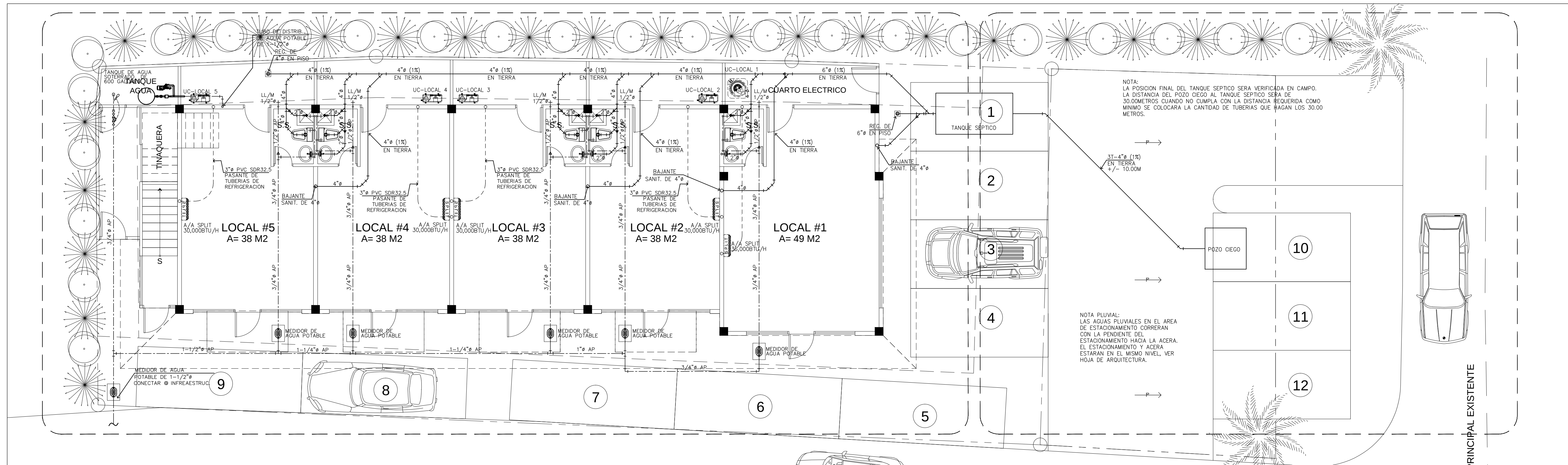
PLANTA GENERAL DE DISTRIBUCION DE PLOMERIA DE NIVEL 000 ESCALA 1:50
