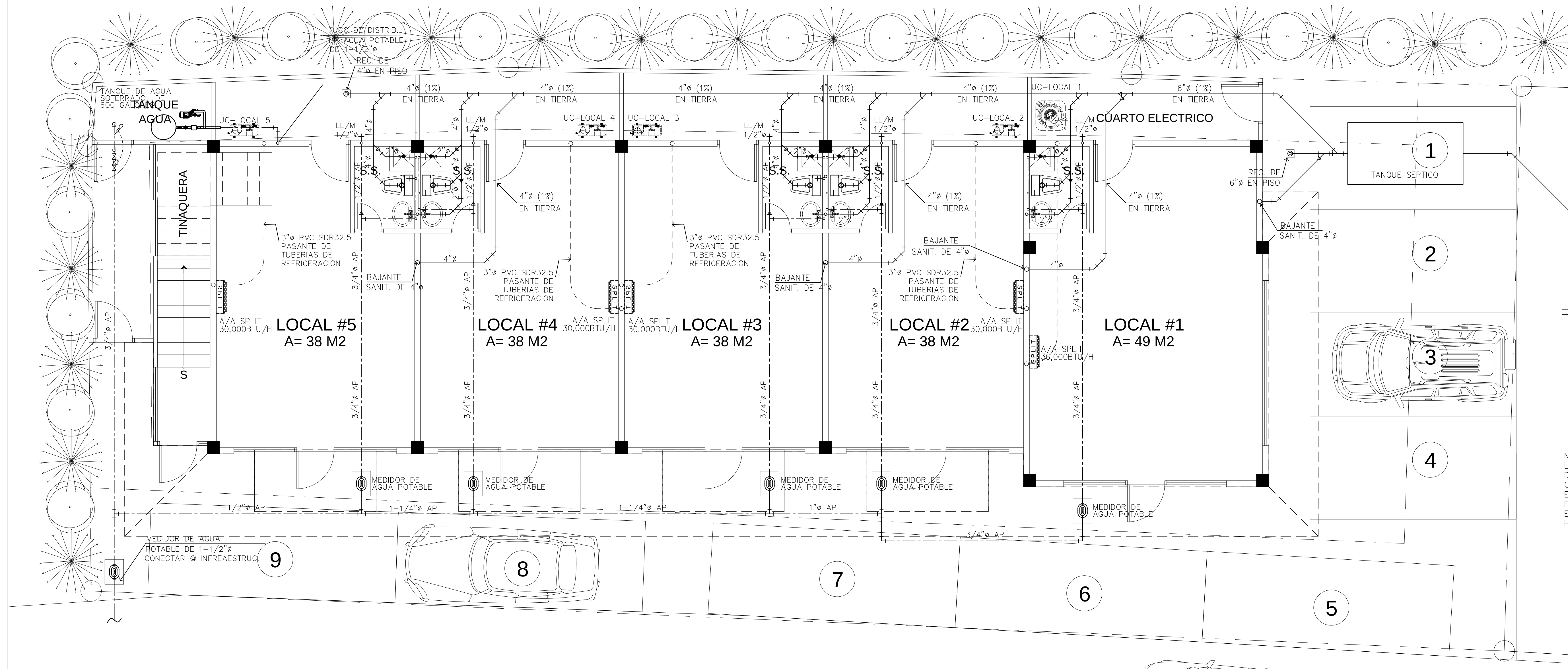
PLANTA DE DISTRIBUCION DE PLOMERIA DE NIVEL 000 (PARTE A) ESCALA 1:50
