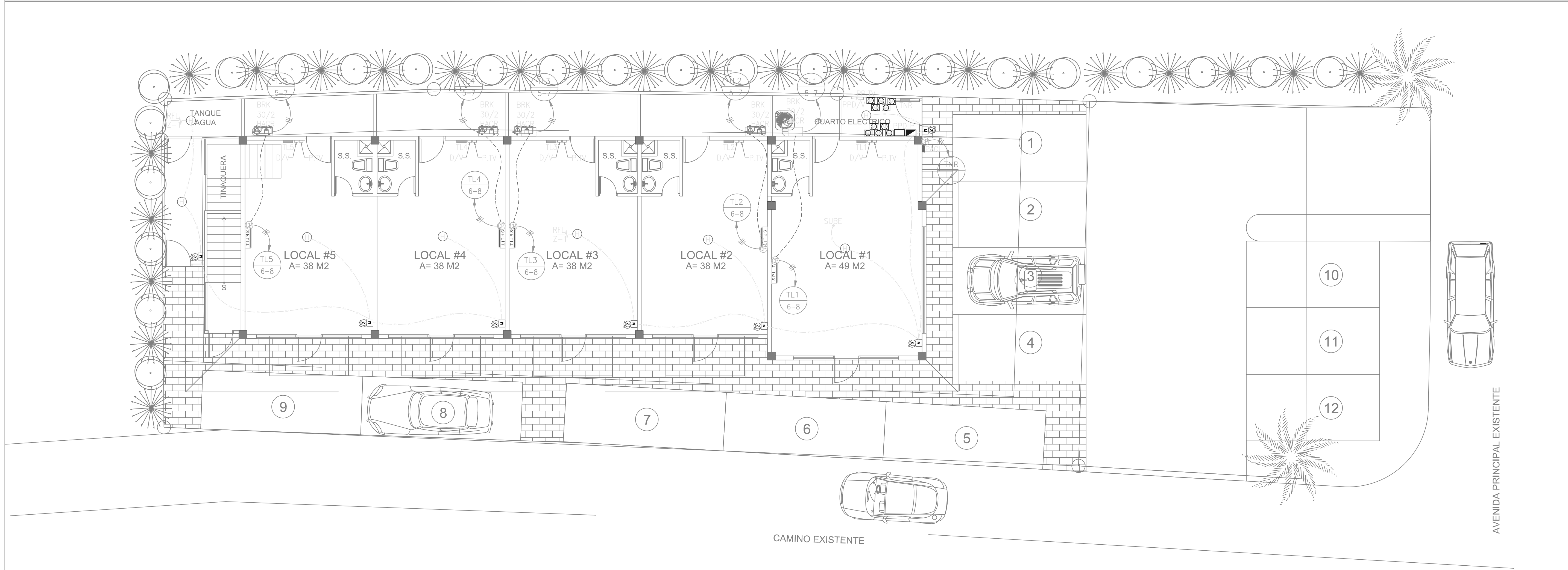
PLANTA DE SISTEMAS ESPECIALES Y A/A NIVEL 000
