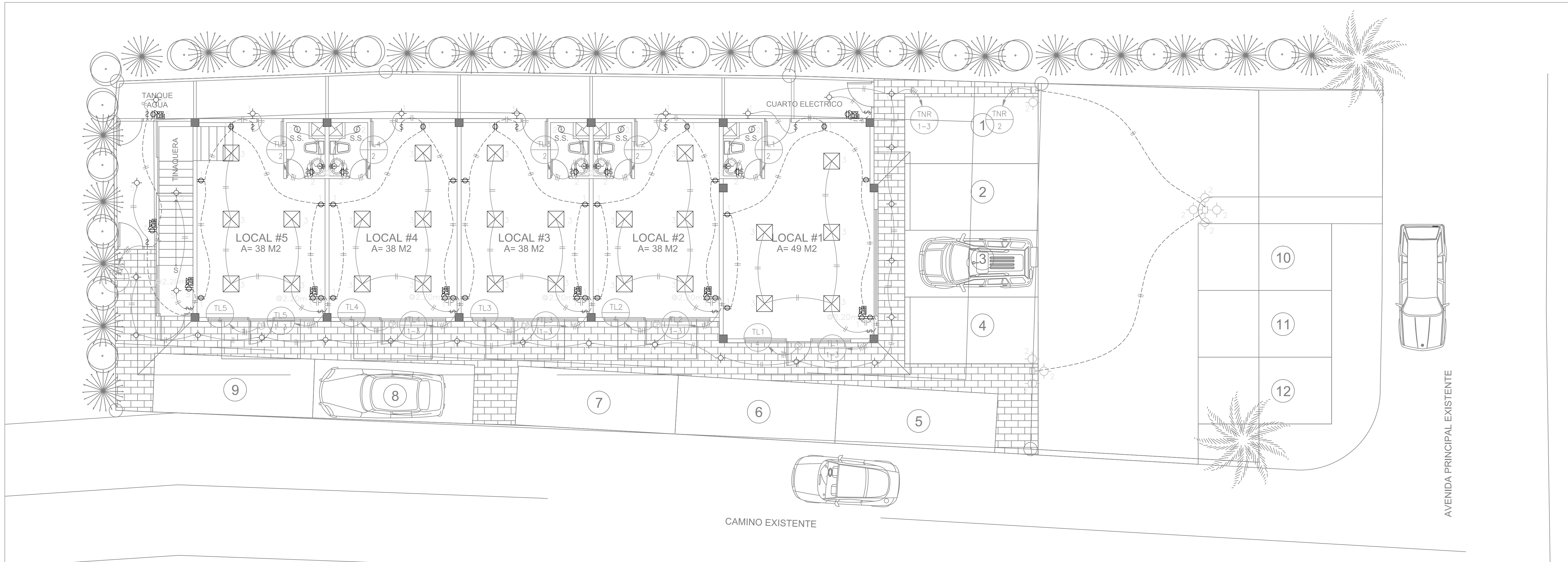
PLANTA DE ILUMINACION Y FUERZA NIVEL 000
