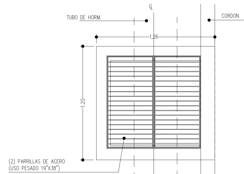
PLANTA DE CAJA PLUVIAL DET.1 ESC. 1: 20
