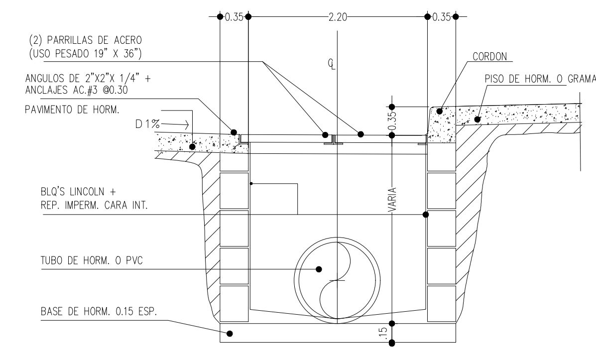
DETALLE CAJA PLUVIAL DET.3 ESC. 1: 20
