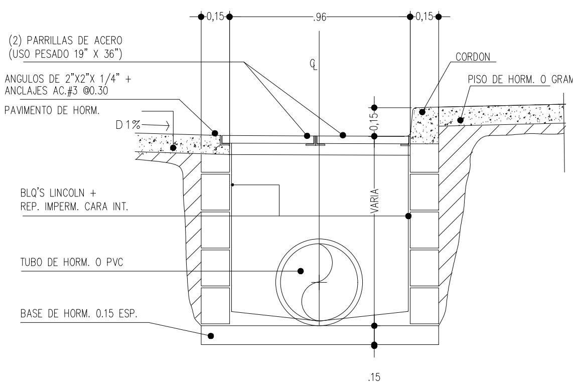
DETALLE CAJA PLUVIAL DET.1 ESC. 1: 20
