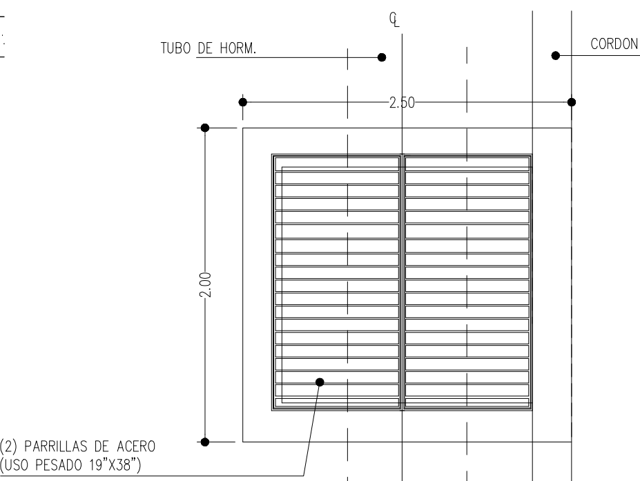
PLANTA DE CAJA PLUVIAL DET.2 ESC. 1: 20
