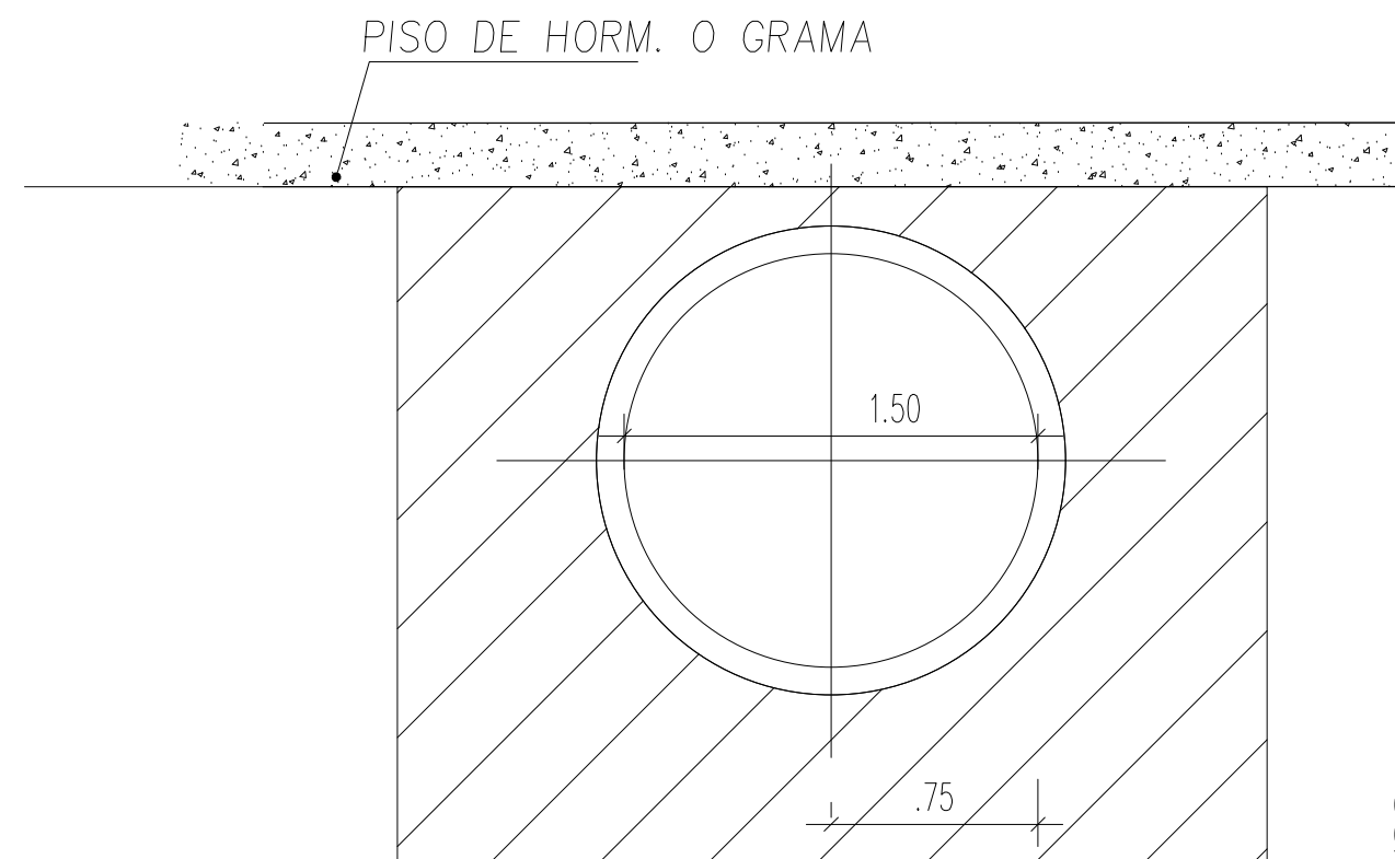
DETALLE CAJA PLUVIAL DET.2 ESC. 1: 50
