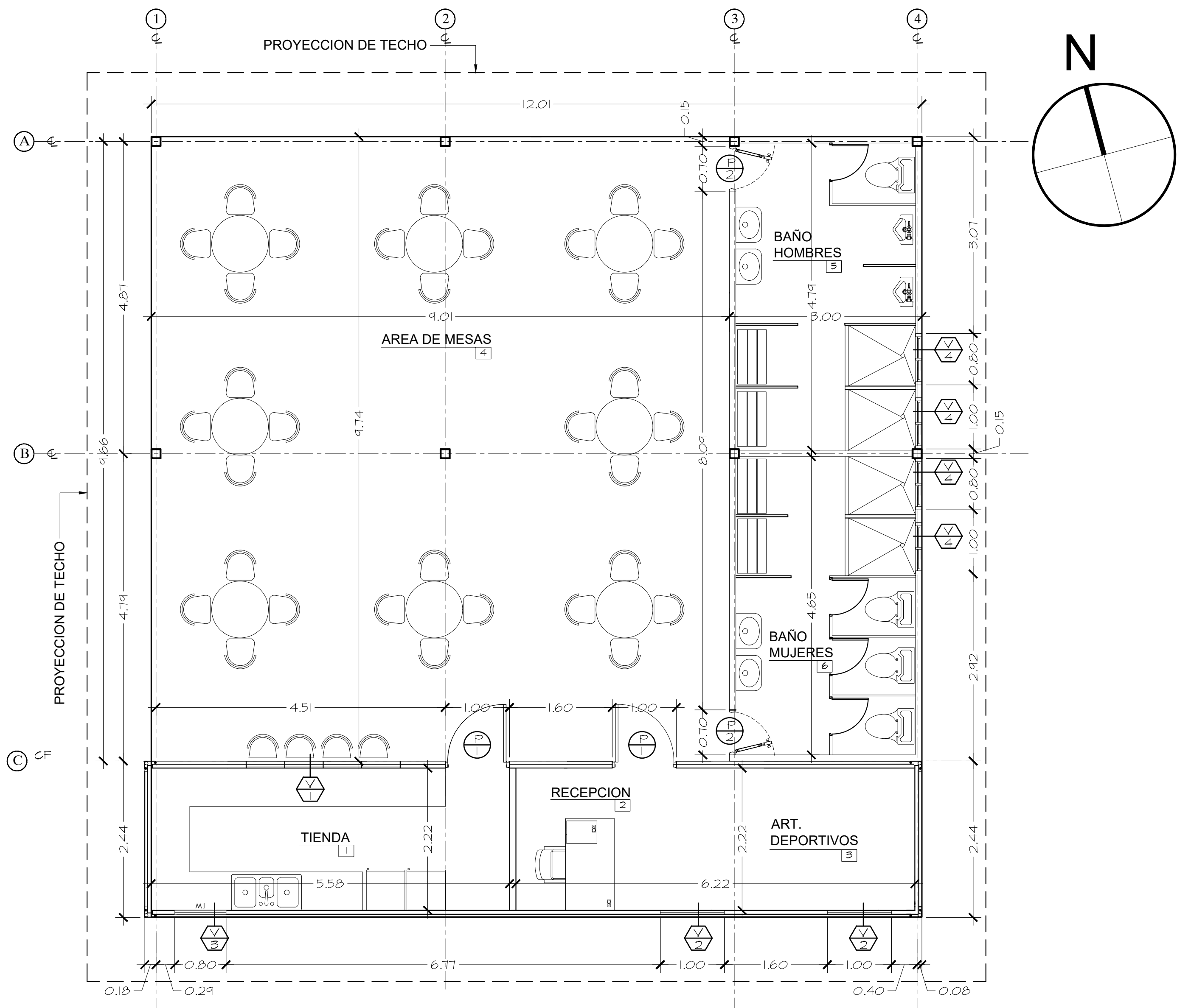
PLANTA ARQUITECTONICA (KIOSCO) ESCALA 1:50
