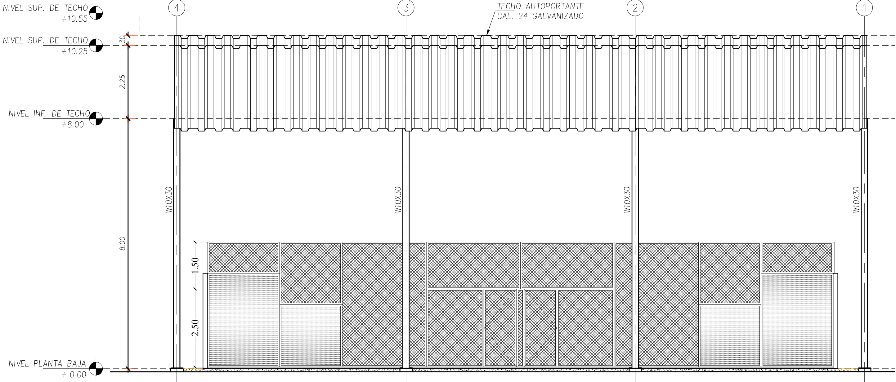
ELEVACION OESTE (CANCHAS) ESCALA 1:75
