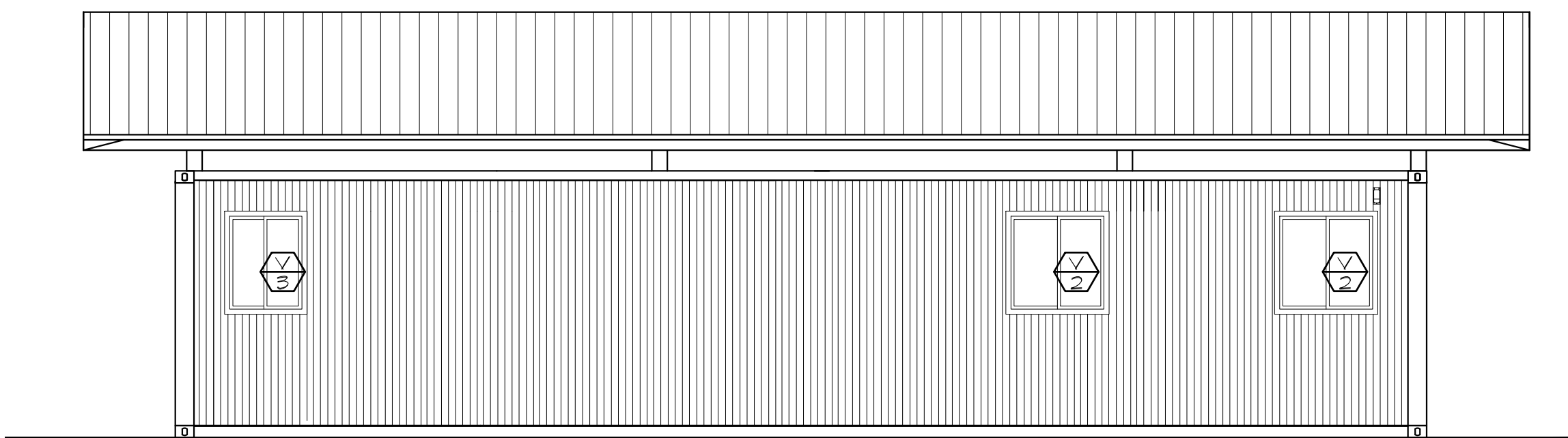
ELEVACION SUR (KIOSCO) ESCALA 1:50
