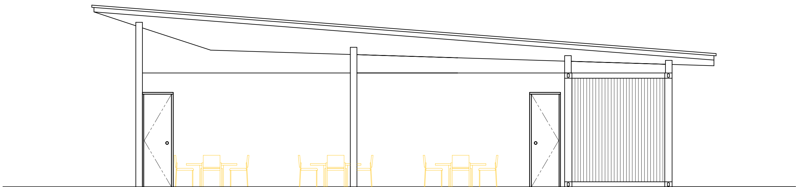
ELEVACION OESTE (KIOSCO) ESCALA 1:50
