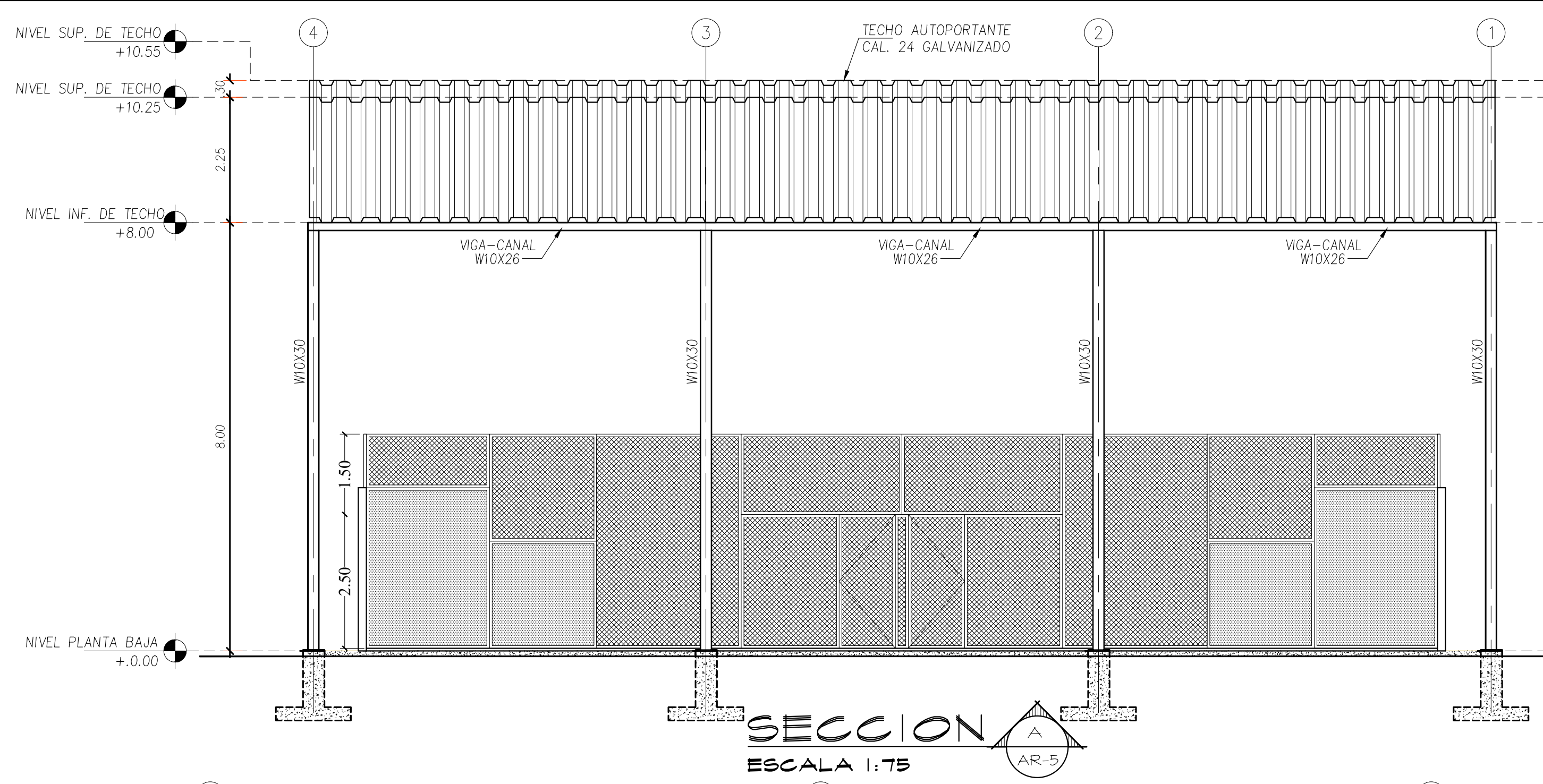
DIMENSIONES CANCHA ESCALA 1:75
