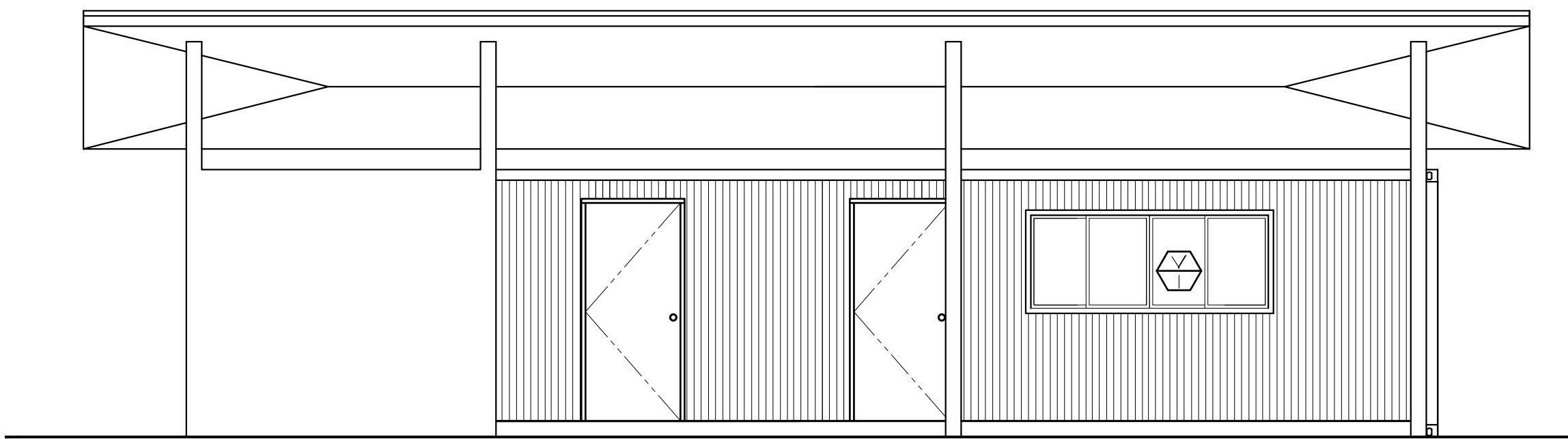
ELEVACION NORTE (KIOSCO) ESCALA 1:50
