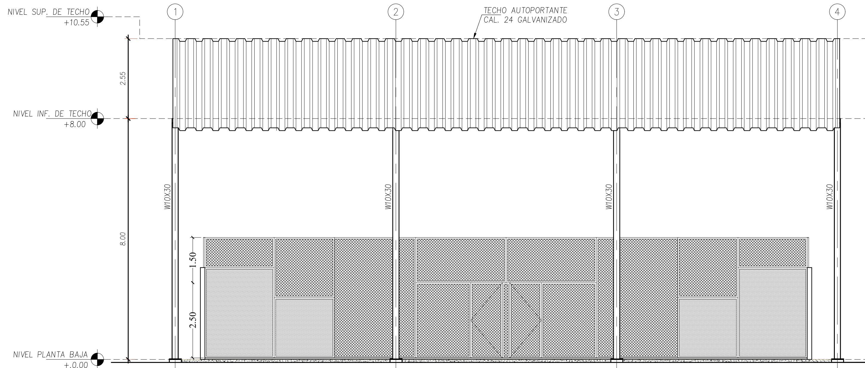
ELEVACION ESTE (CANCHAS) ESCALA 1:75
