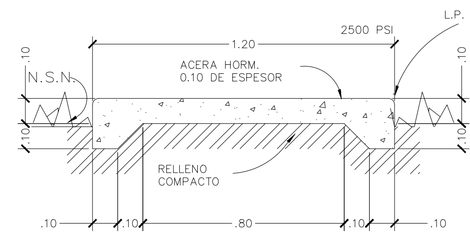
DET. TIPO DE ACERA ESCALA 1:15
