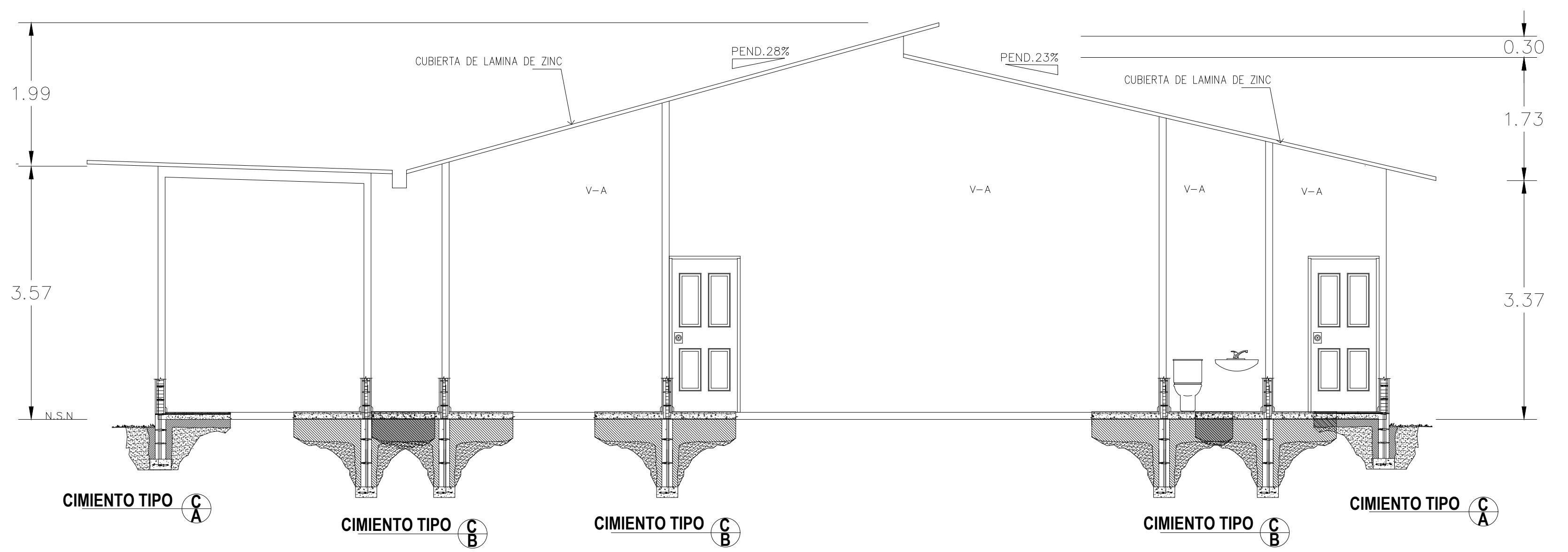
SECCION N°1 ESCALA: 1:50
