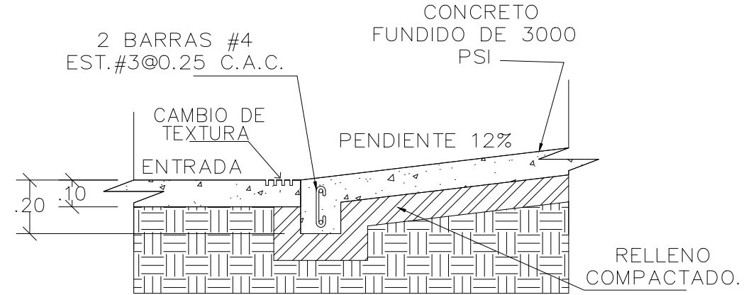
DET. ACERA-RAMPA DISCAPACITADOS ESC.1:20
