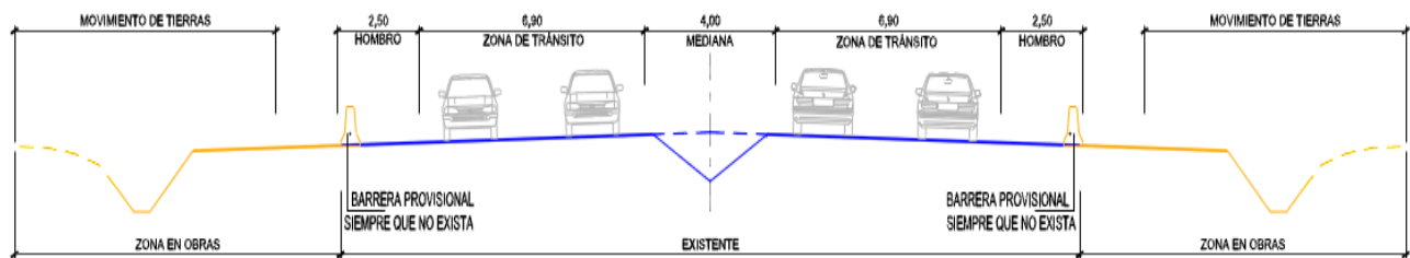
Ilustración 6 - Ampliación por ambos márgenes - Etapa 1
