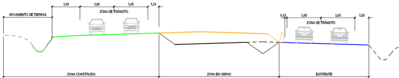
Ilustración 19 - Corrección de curvas en planta - Etapa 2
