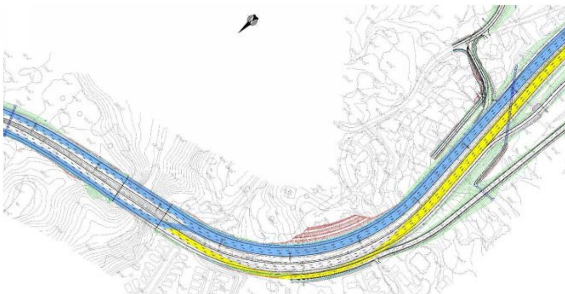
Ilustración 39 – Rectificación de curva Est 52+400 a 53+000
