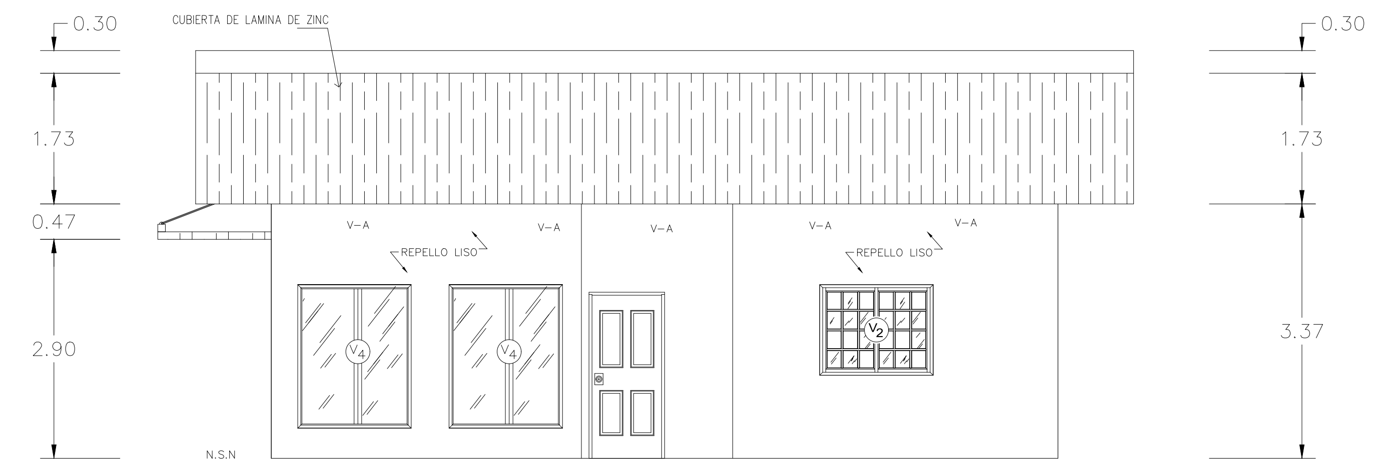
ELEVACION LATERAL IZQUIERDO ESCALA: 1:50
