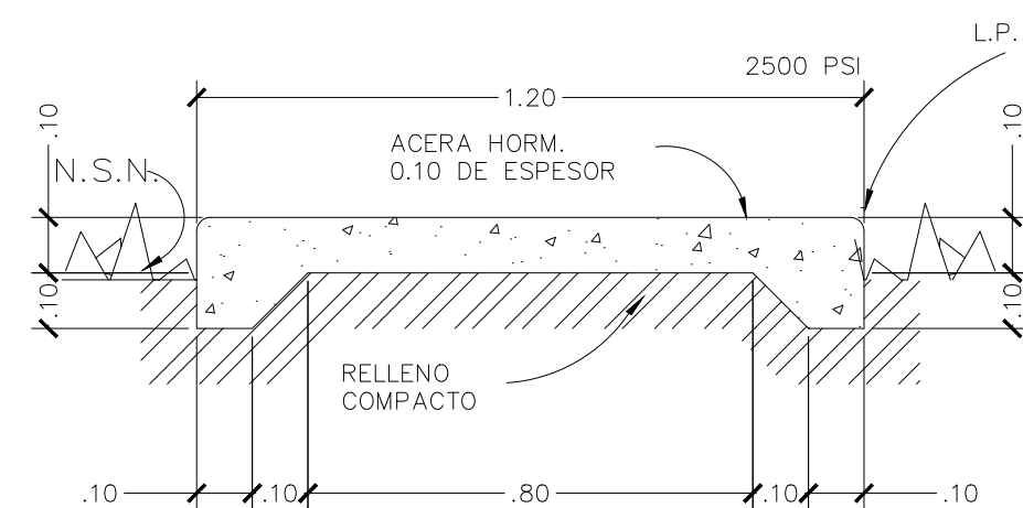
SECCION N°1 ESCALA: 1:50
