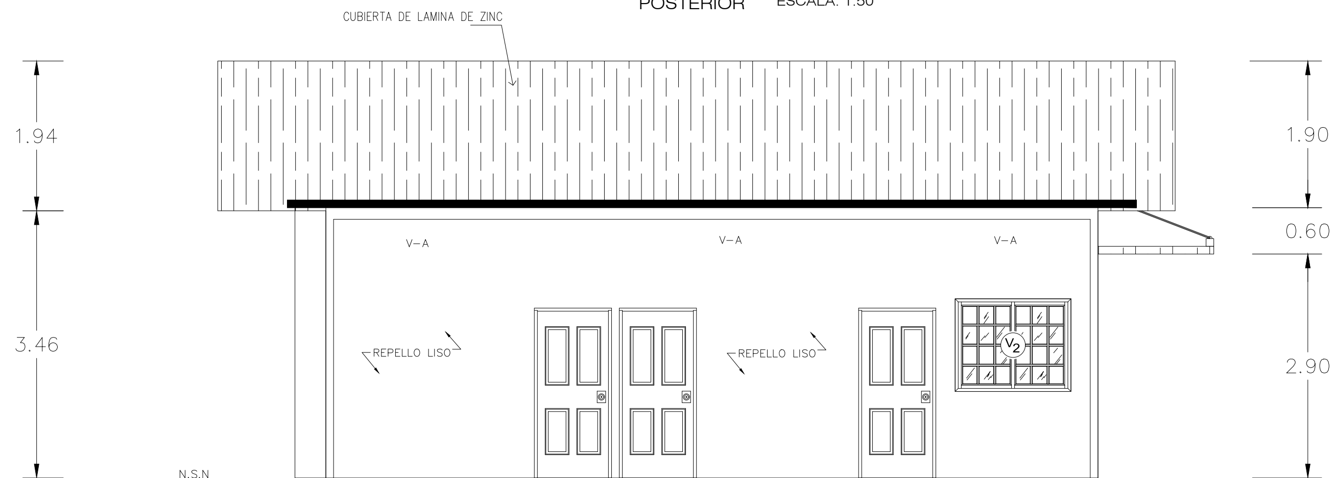
ELEVACION POSTERIOR ESCALA: 1:50
