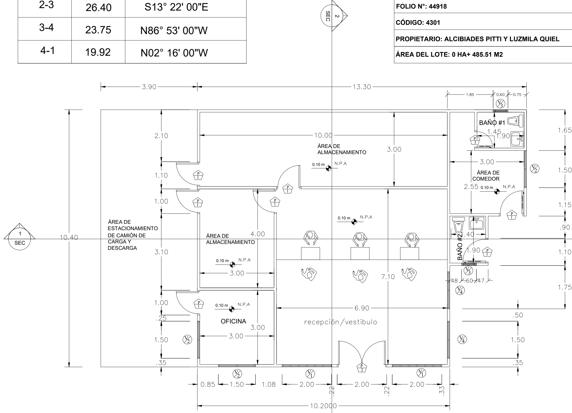
PLANTA ARQUITECTONICA ESCALA: 1:75
