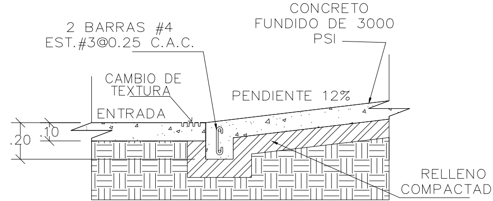
DET. ACERA-RAMPA DISCAPACITADOS ESC.1:20
