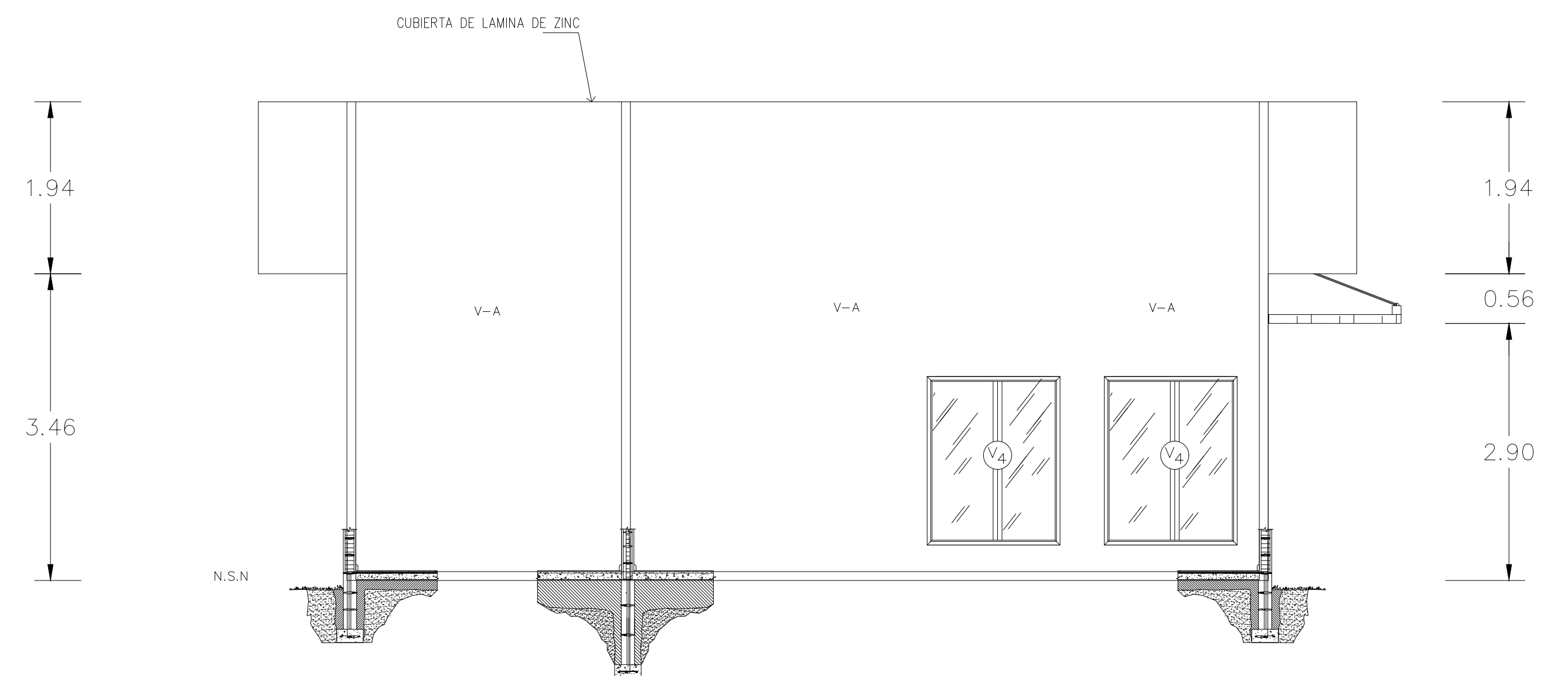
SECCION N°2 ESCALA: 1:50
