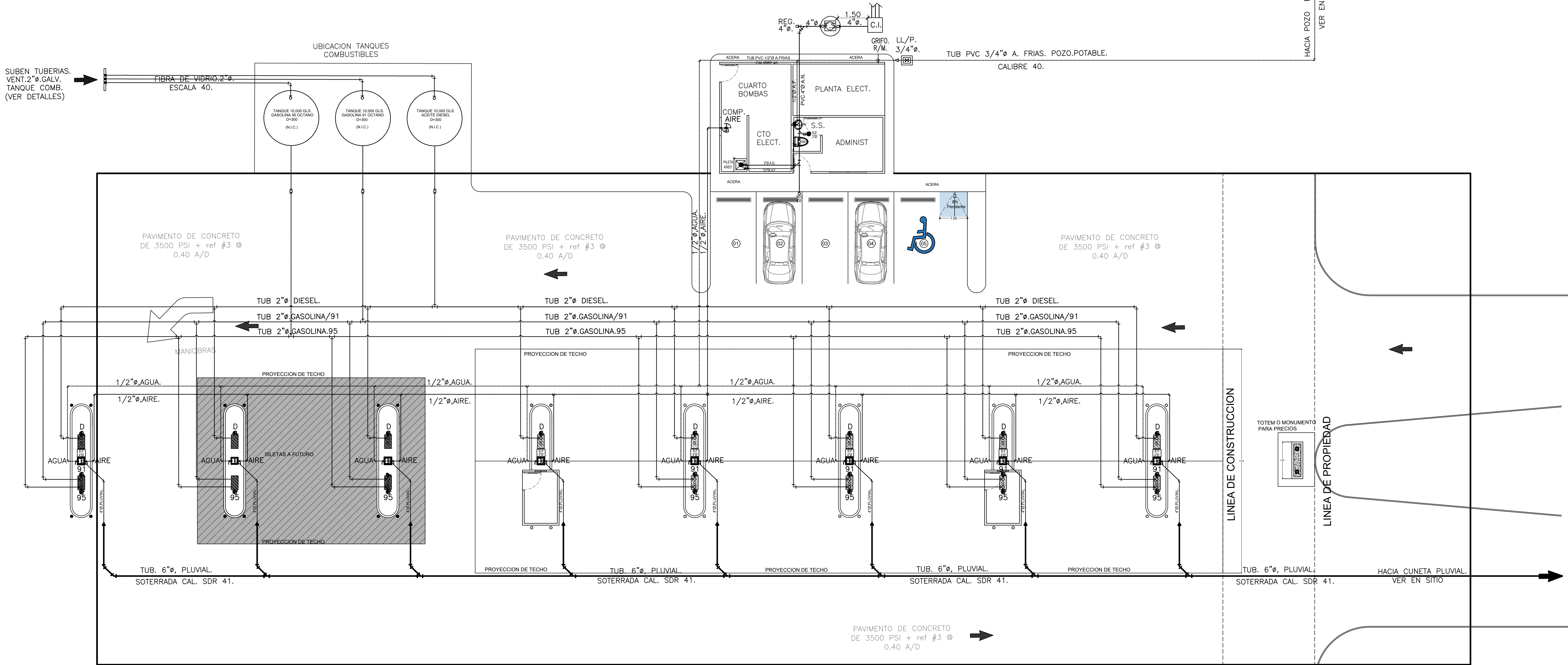
PLANTA GENERAL DE PLOMERIA ESC 1:50
