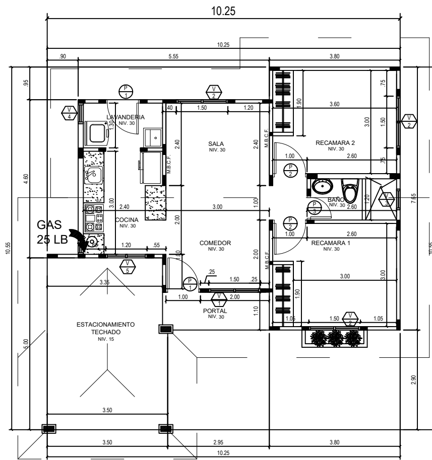
PLANTA ARQUITECTÓNICA ESC. 1:50
