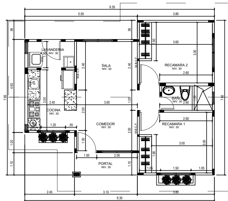
PLANTA ARQUITECTÓNICA ESC. 1:75
