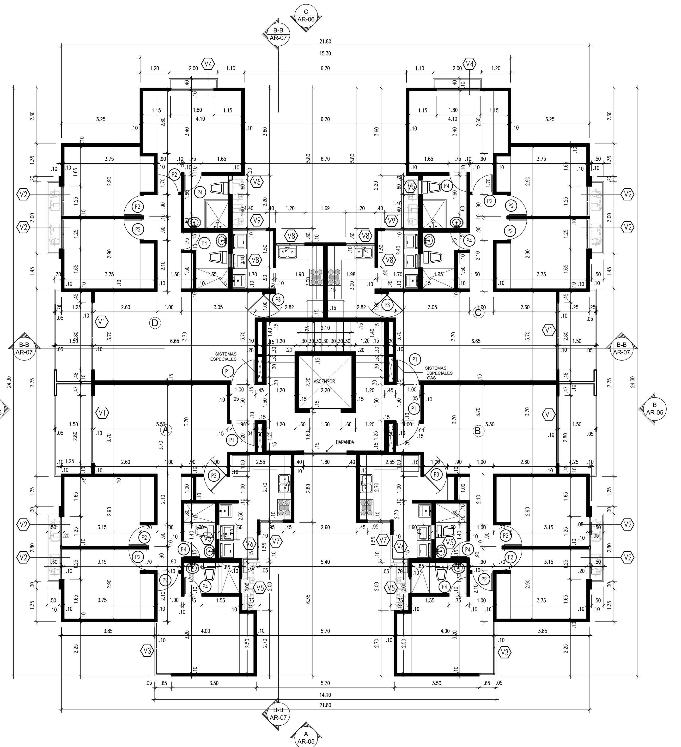
PLANTA NIVEL 700 & 800 ESCALA 1:75
