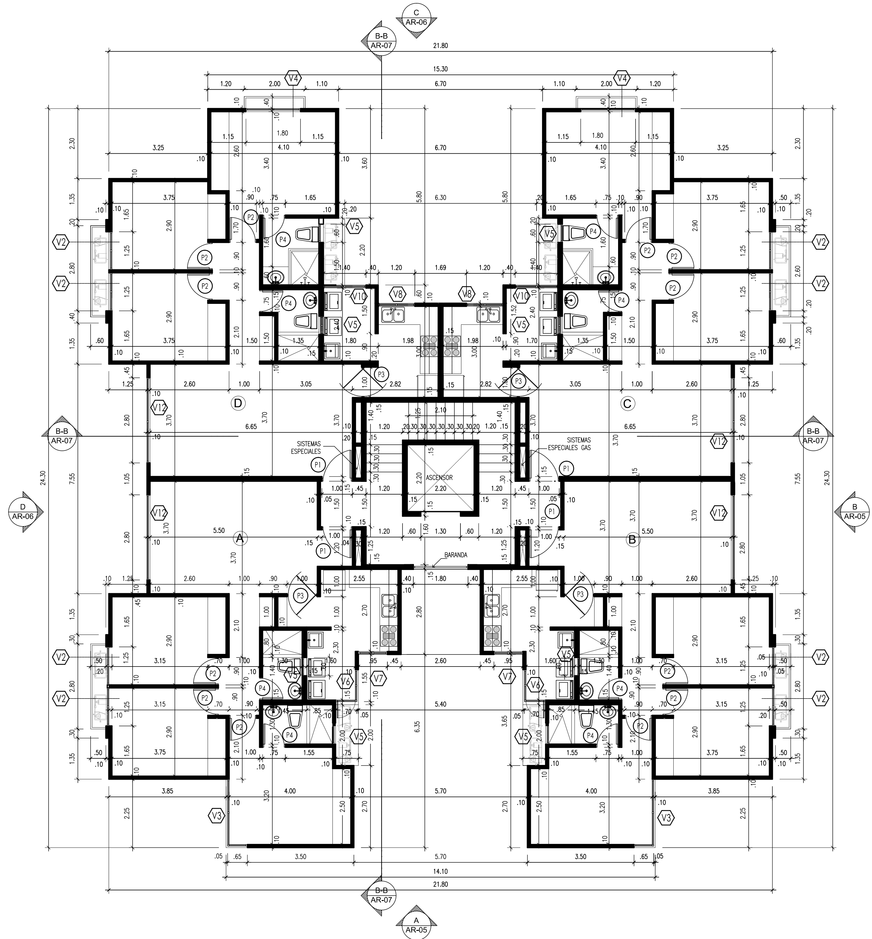
PLANTA NIVEL 200@600 ESCALA 1:75
