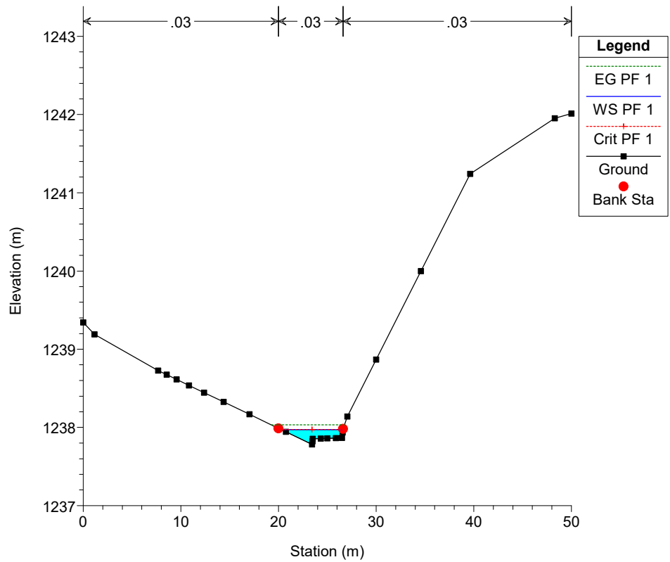
EH QBA SIN NOMBRE VOLCANCITO Plan: PLAN 1 A 50 11/22/2021
