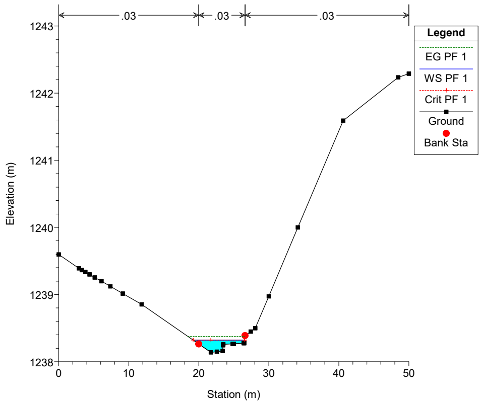
EH QBA SIN NOMBRE VOLCANCITO Plan: PLAN 1 A 50 11/22/2021
