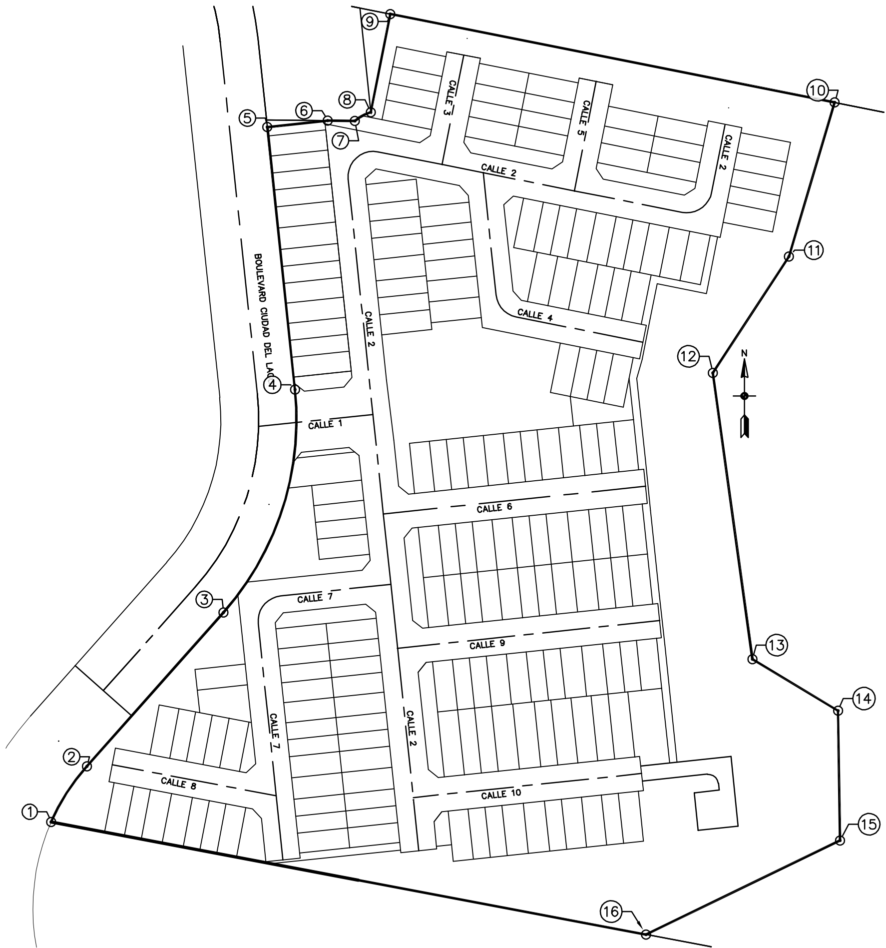
COORDENADAS DE P.H. RIBERAS DEL LAGO ESC. 1:1500 DATUM WGS-84
