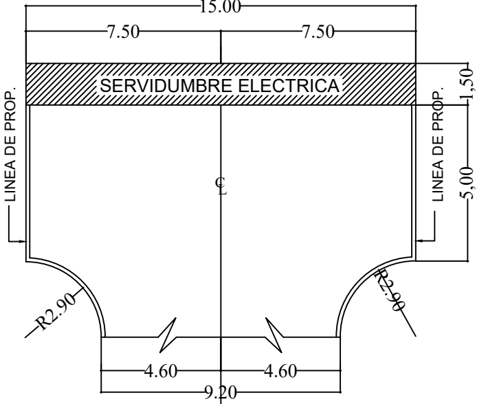
DETALLE DE MARTILLO ESCALA 1/200
