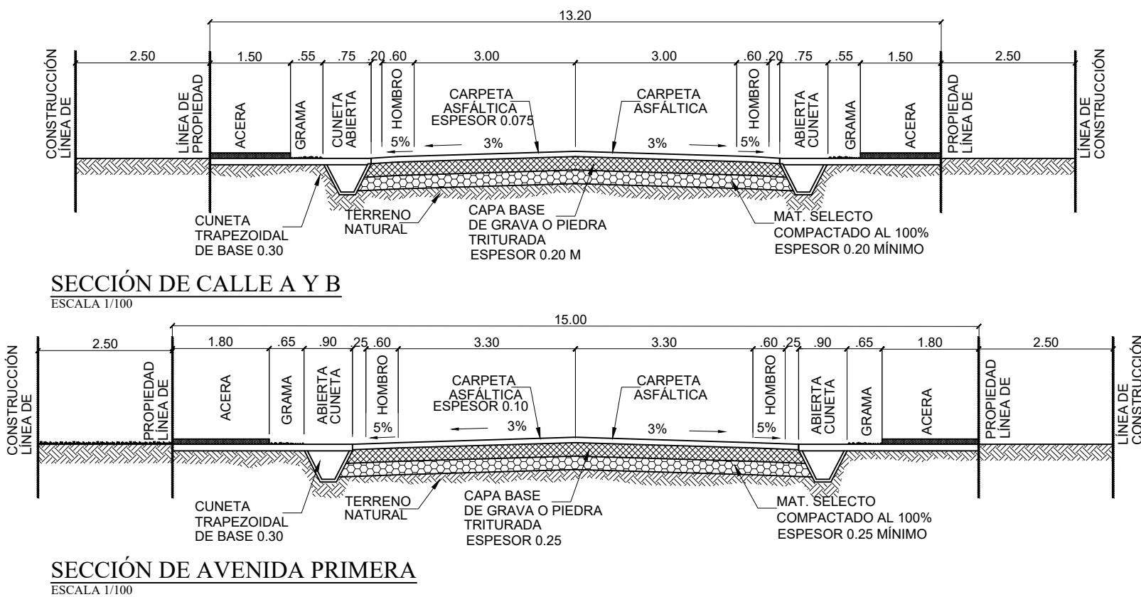
SECCIÓN DE AVENIDA PRIMERA ESCALA 1/100
