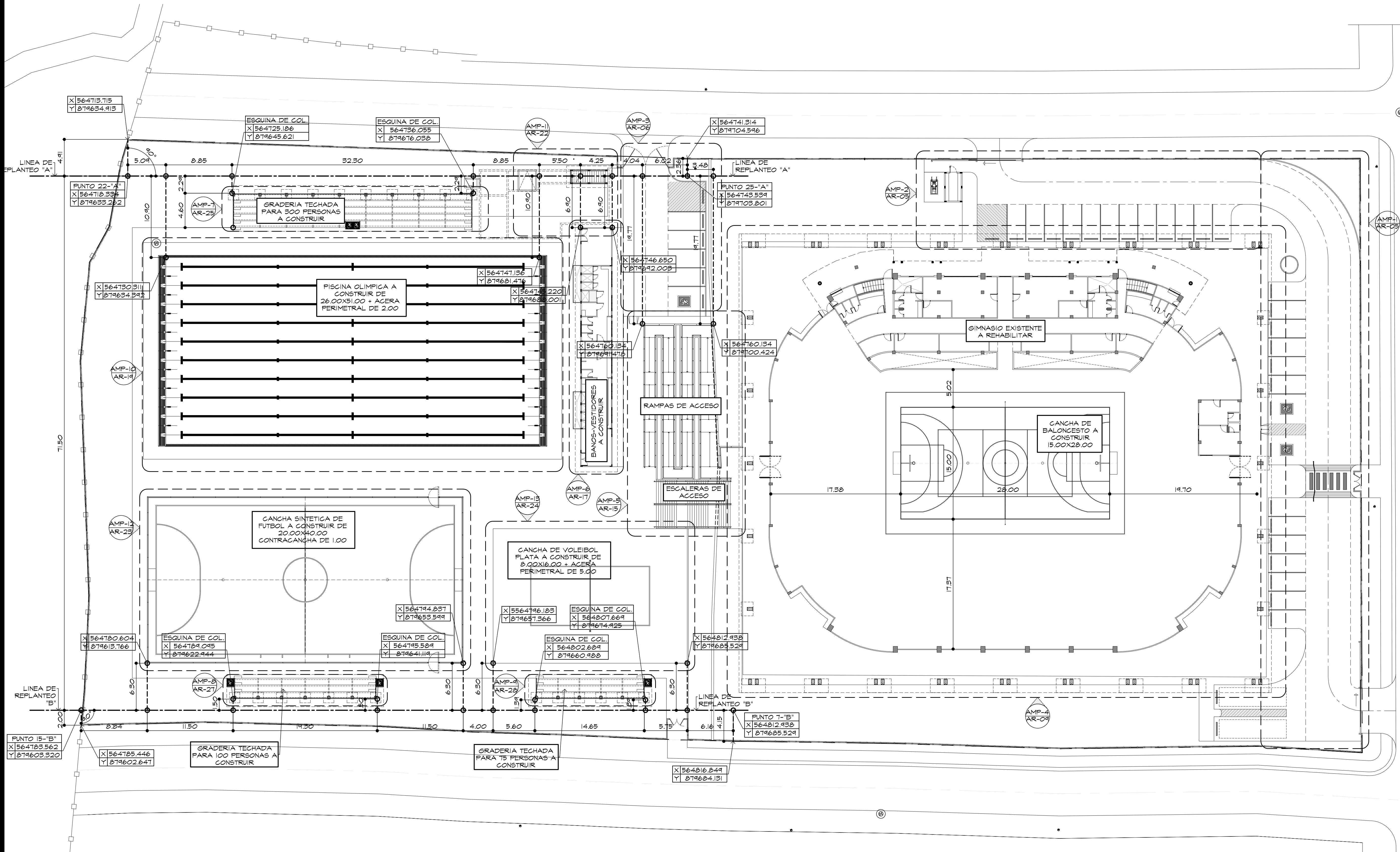
PLANTA GENERAL DE NUEVA ARQUITECTURA DE REPLANTEO- NIVEL 000 ESC. 1/ 250
