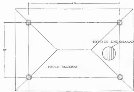
PLANTA DE GAZEBO
