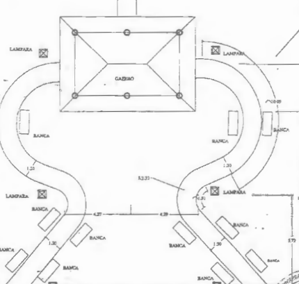
PLANTA DE GAZEBO Y PARQUE
