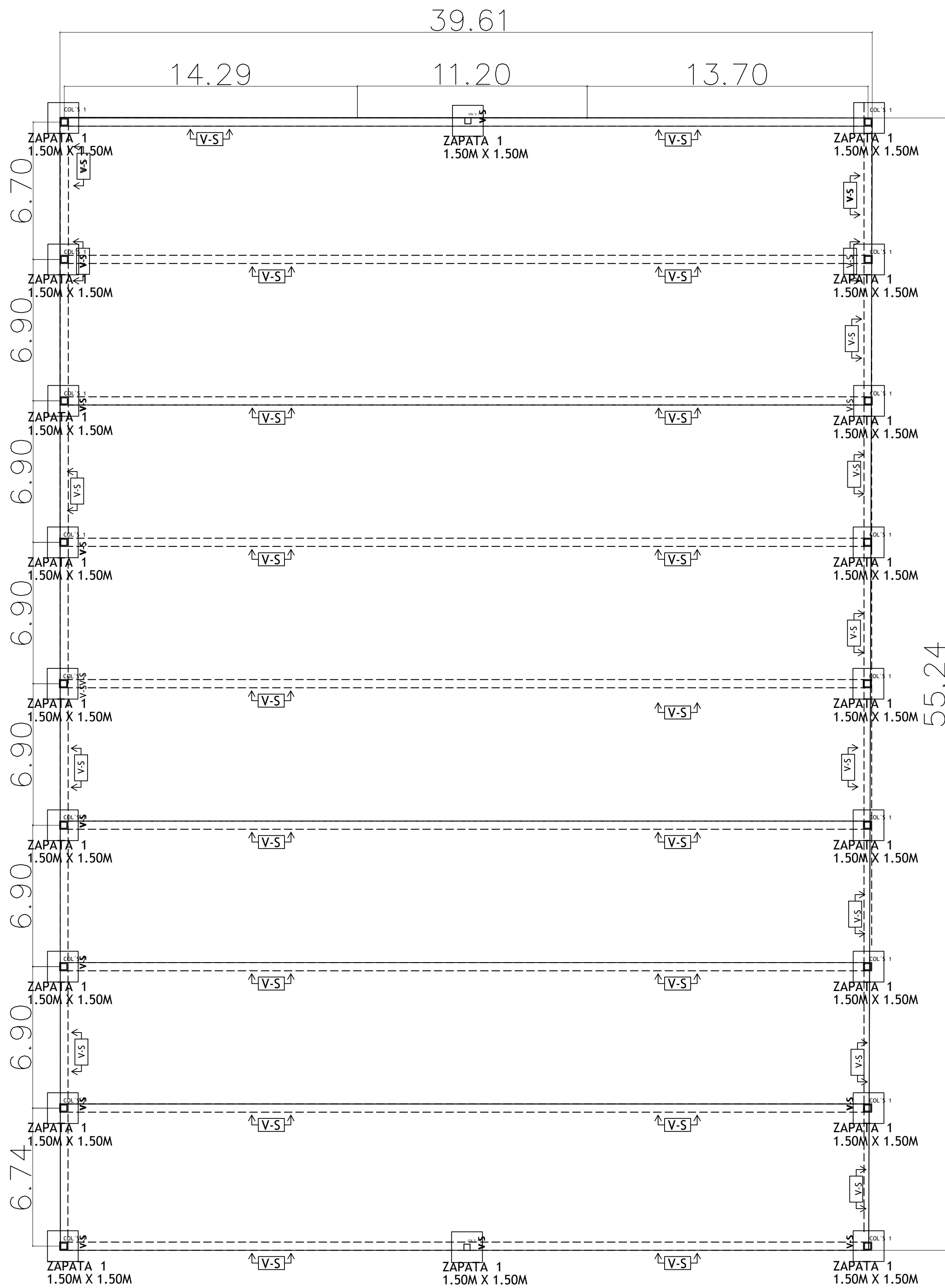
PLANTA DE ZAPATAS
