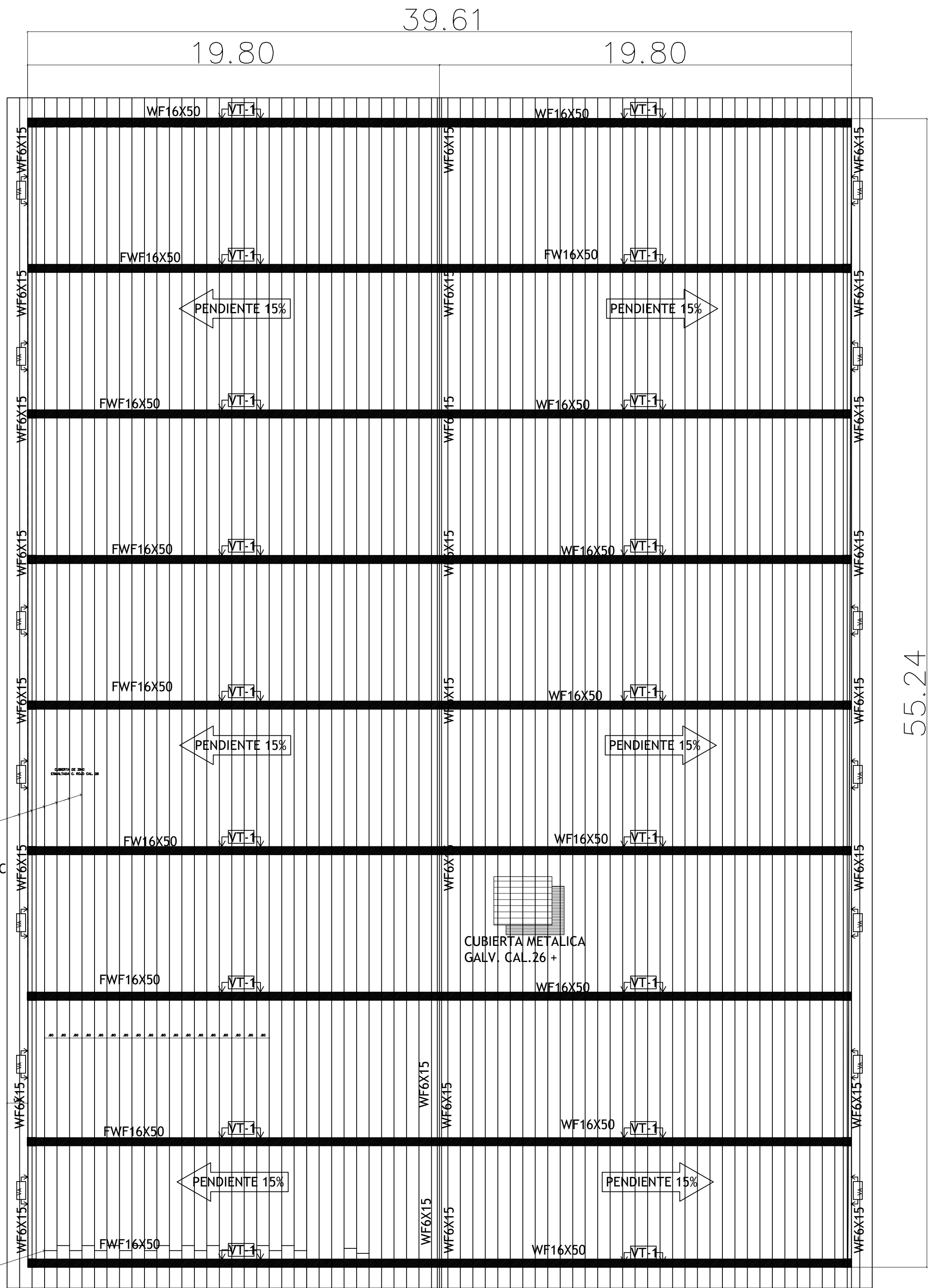
PLANTA DE TECHO
