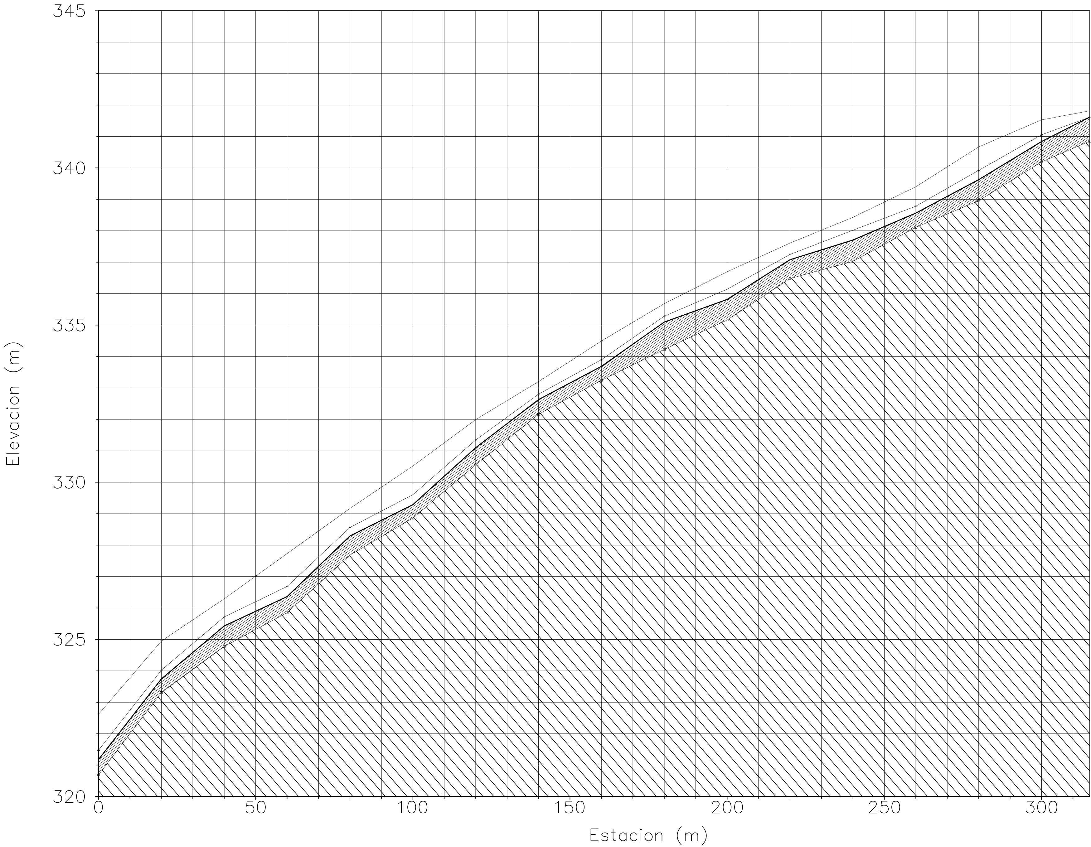
PLANO-PERFIL DE QUEBRADA SIN NOMBRE
