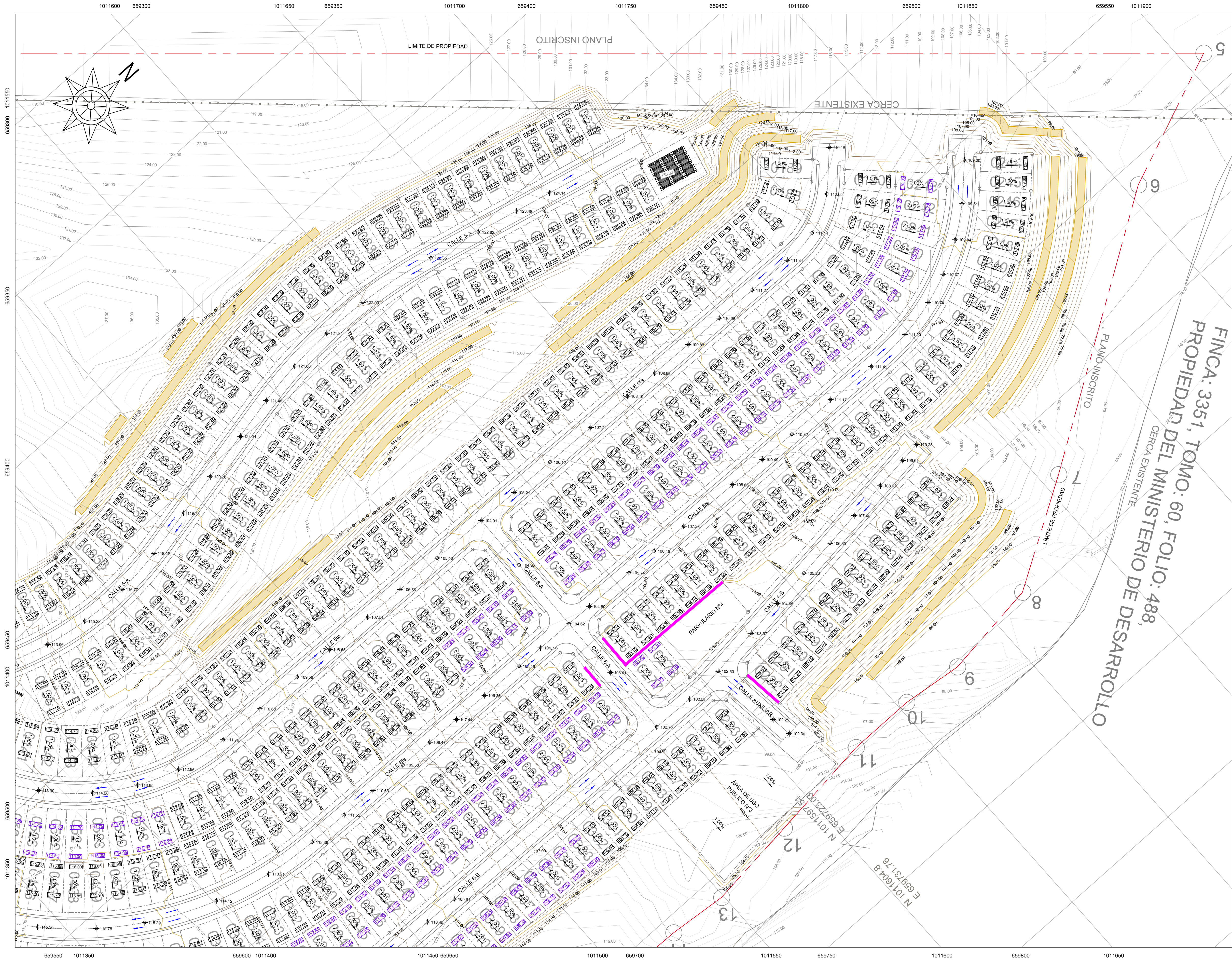
PLANTA DE TERRACERÍA - HOJA 02 ESCALA 1:750
