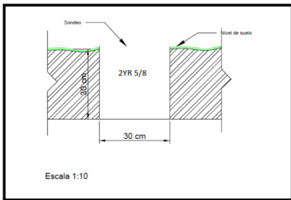
Ilustración 8.4. 4: estratigrafía sondeos
