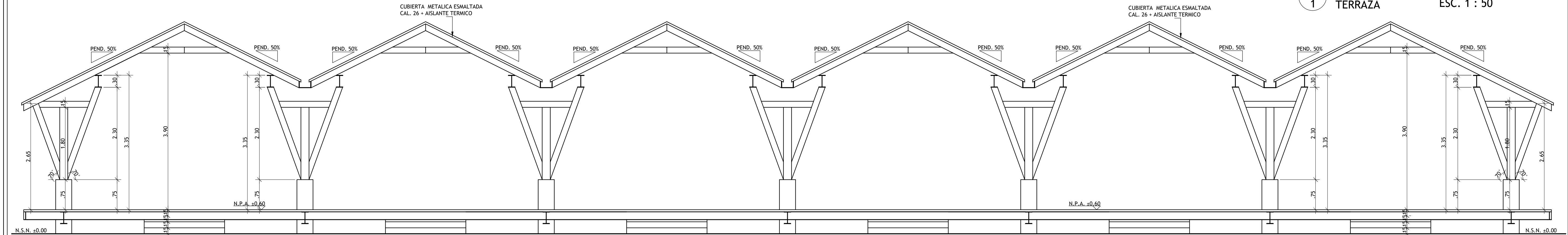
E 3 ELEVACION POSTERIOR TERRAZA ESC. 1 : 50
