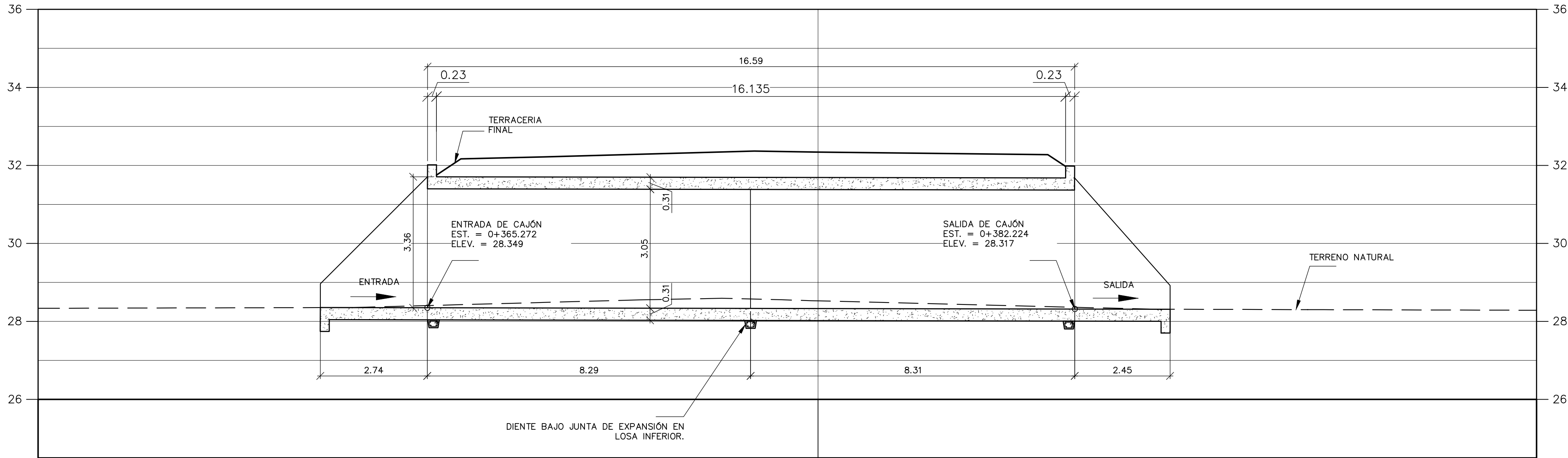
PERFIL DEL CAJON ESC. 1:75
