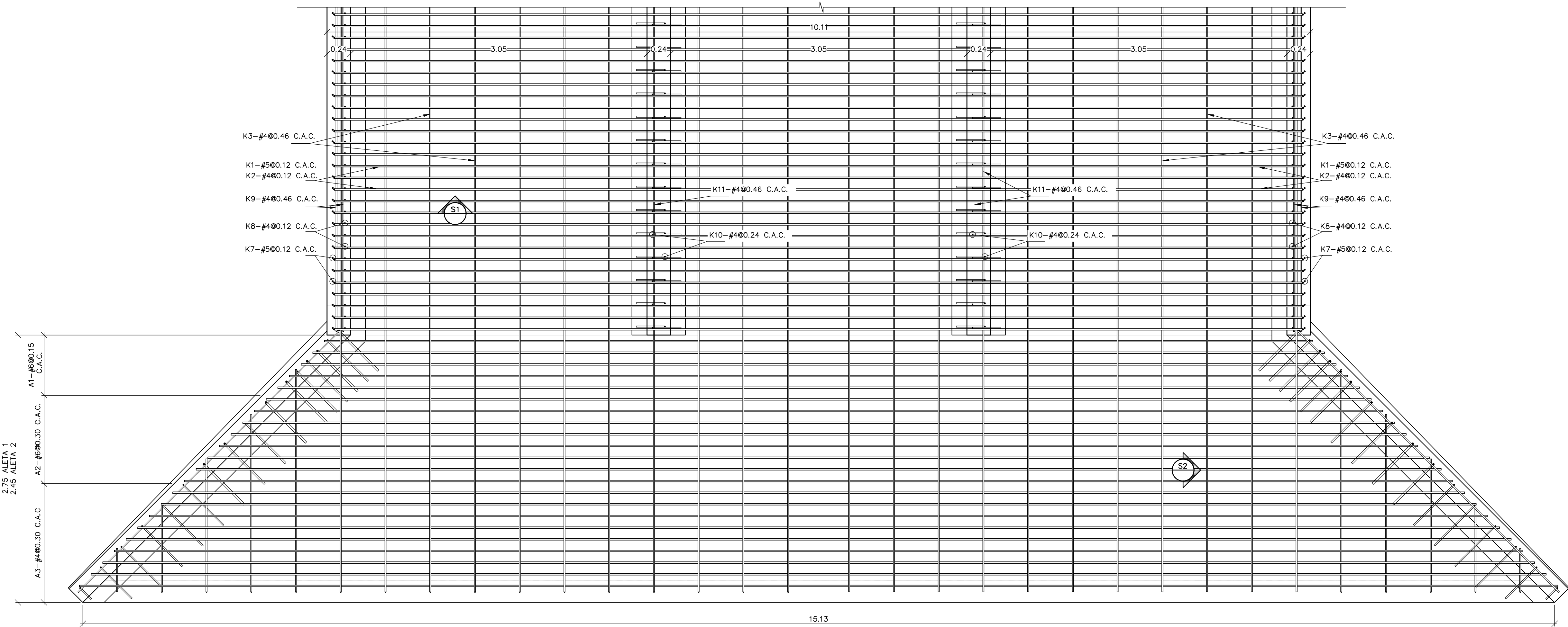
PLANTA ESTRUCTURAL DE LOSA DE CAJON ESC. 1:25
