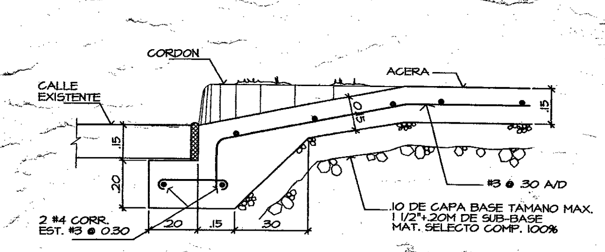
DETALLE DE EMPALME DE LOSA ESCALA 1:15
