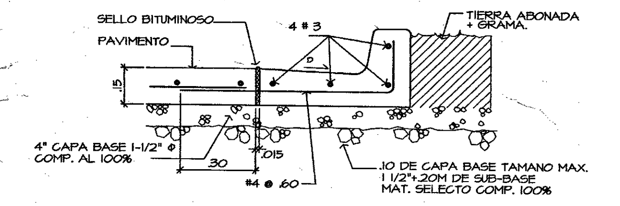
DETALLE DE CORDON ESCALA 1:15
