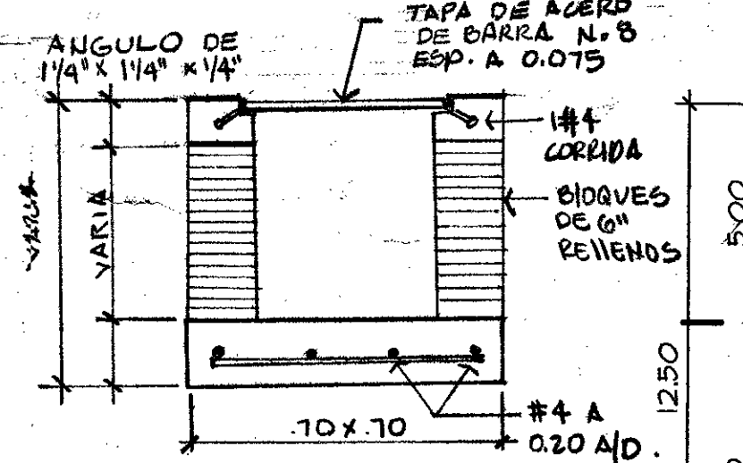
DETALLE DE MEDIA CANA (DONDE SE REQUIERA) ESCALA 1:15
