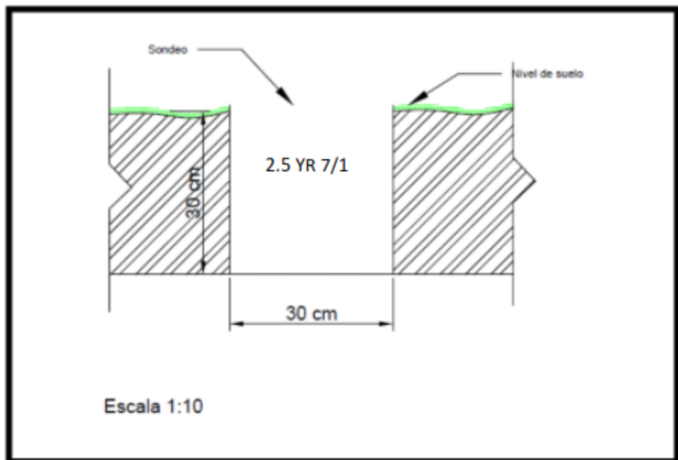
Ilustración 8.4. 4: estratigrafía sondeos
