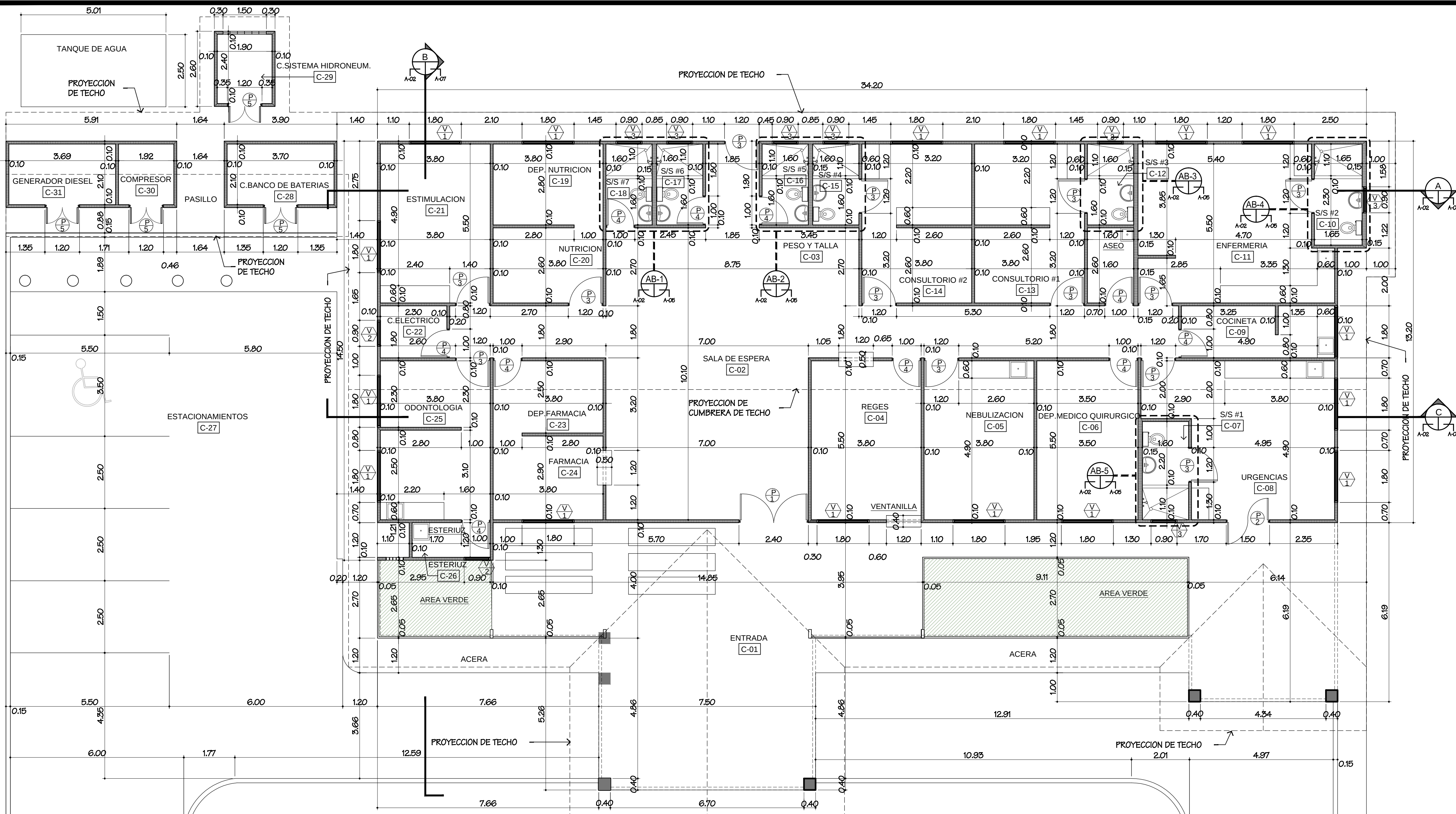
PLANTA ARQUITECTONICA CENTRO DE SALUD ESC. 1:75
