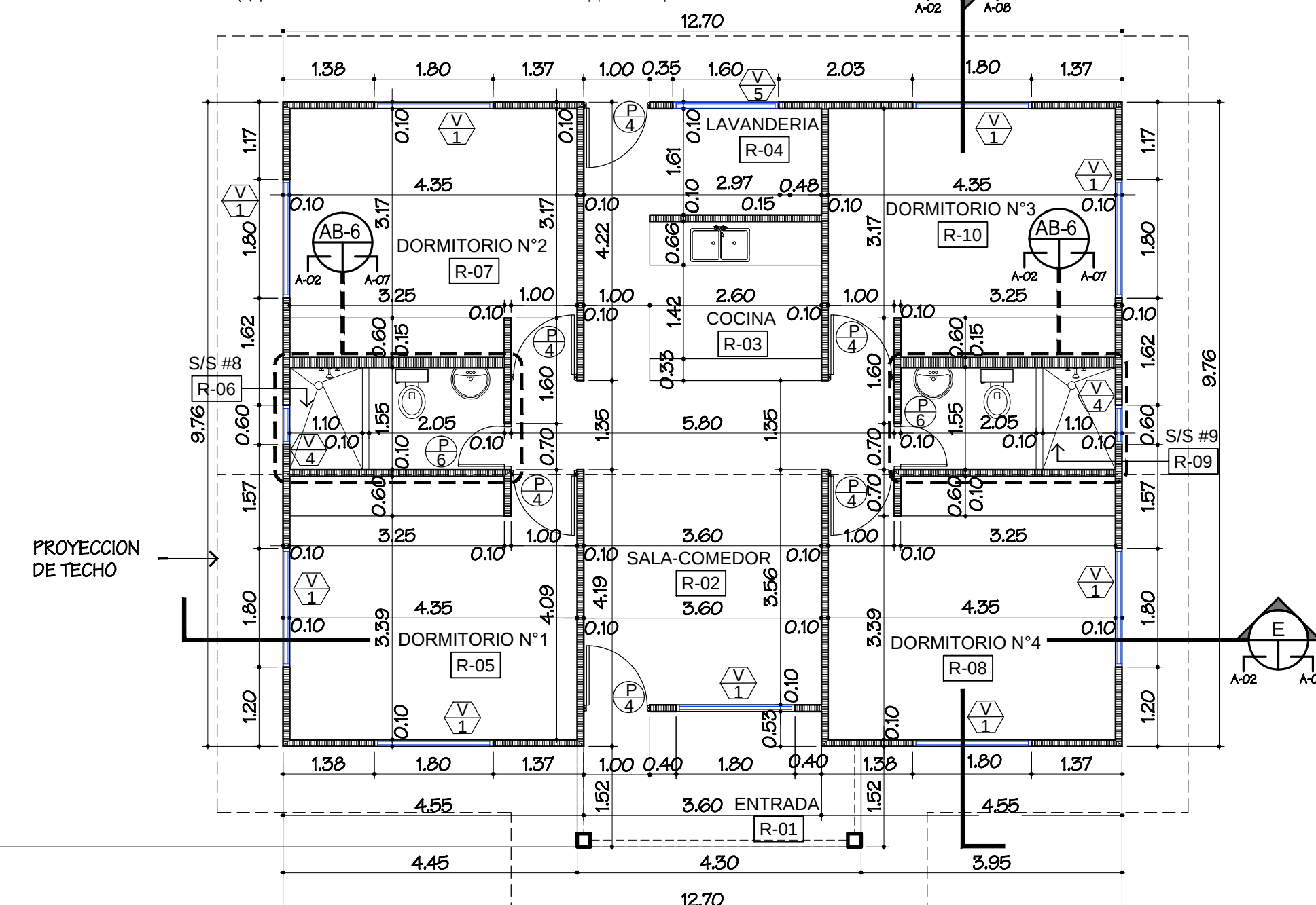
PLANTA ARQUITECTONICA RESIDENCIA FUNCIONARIOS ESC. 1:75
