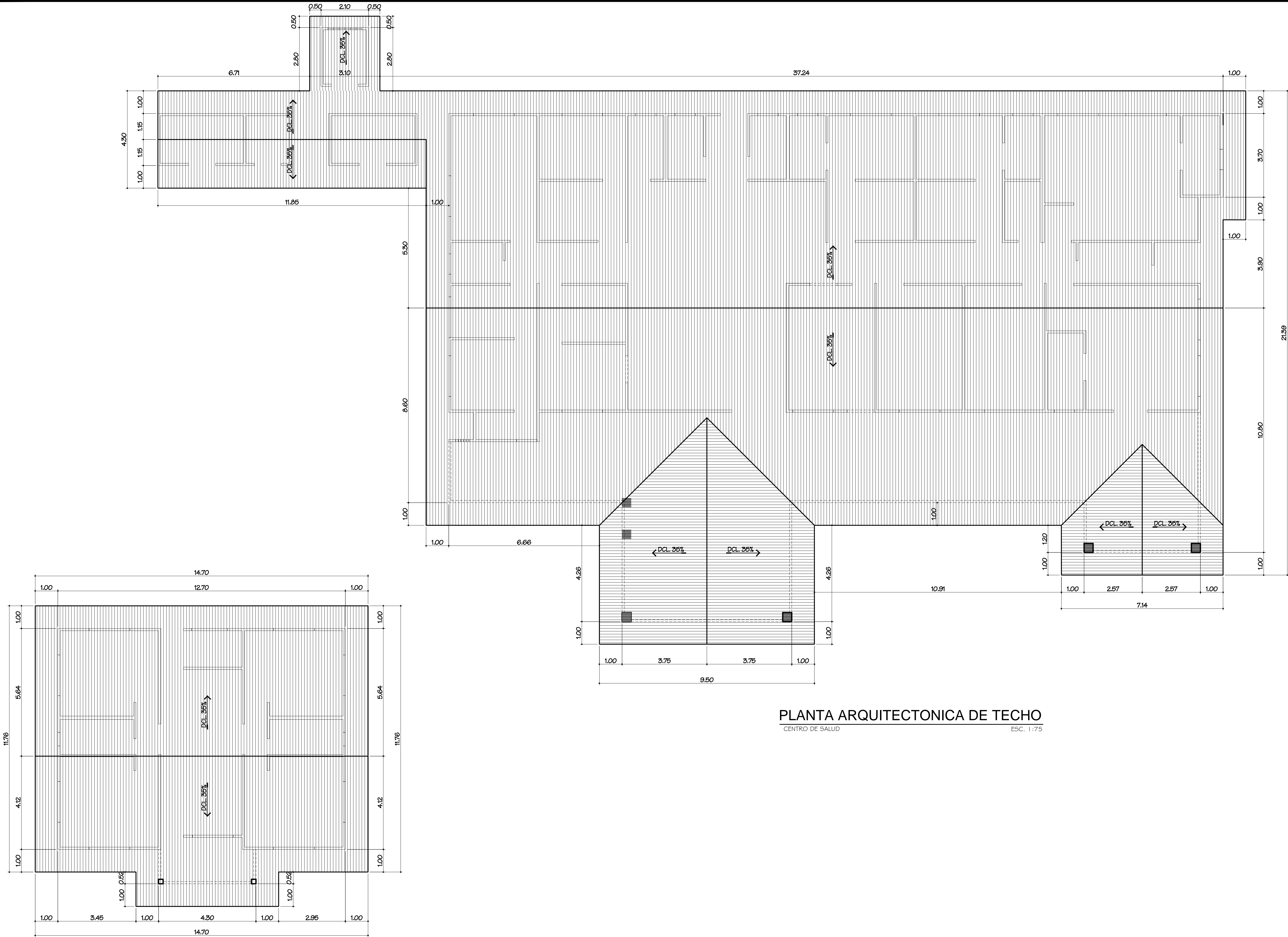
PLANTA ARQUITECTONICA DE TECHO RESIDENCIA FUNCIONARIOS ESC. 1:75
