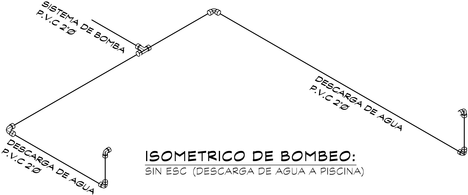
ISOMETRICO DE BOMBEO: SIN ESC (SUCCION SKIMMER)
