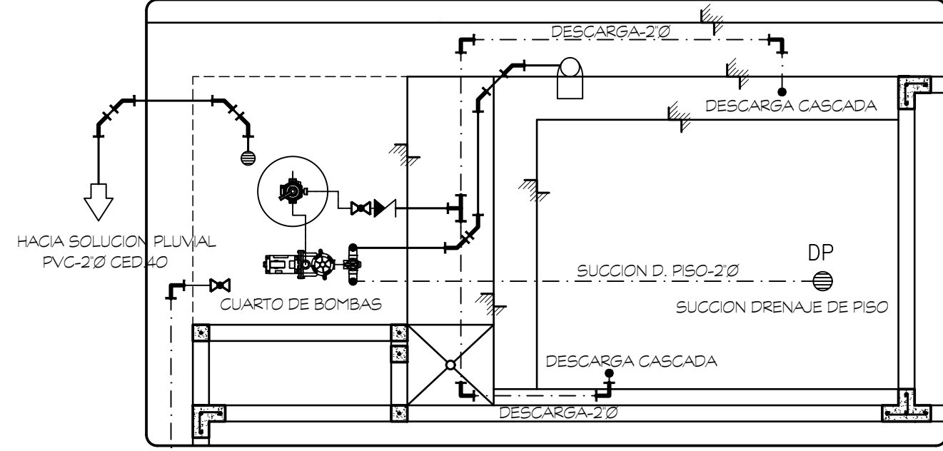
PLANTA DE PLOMERIA: ESC: 1:50 (PISCINA)
