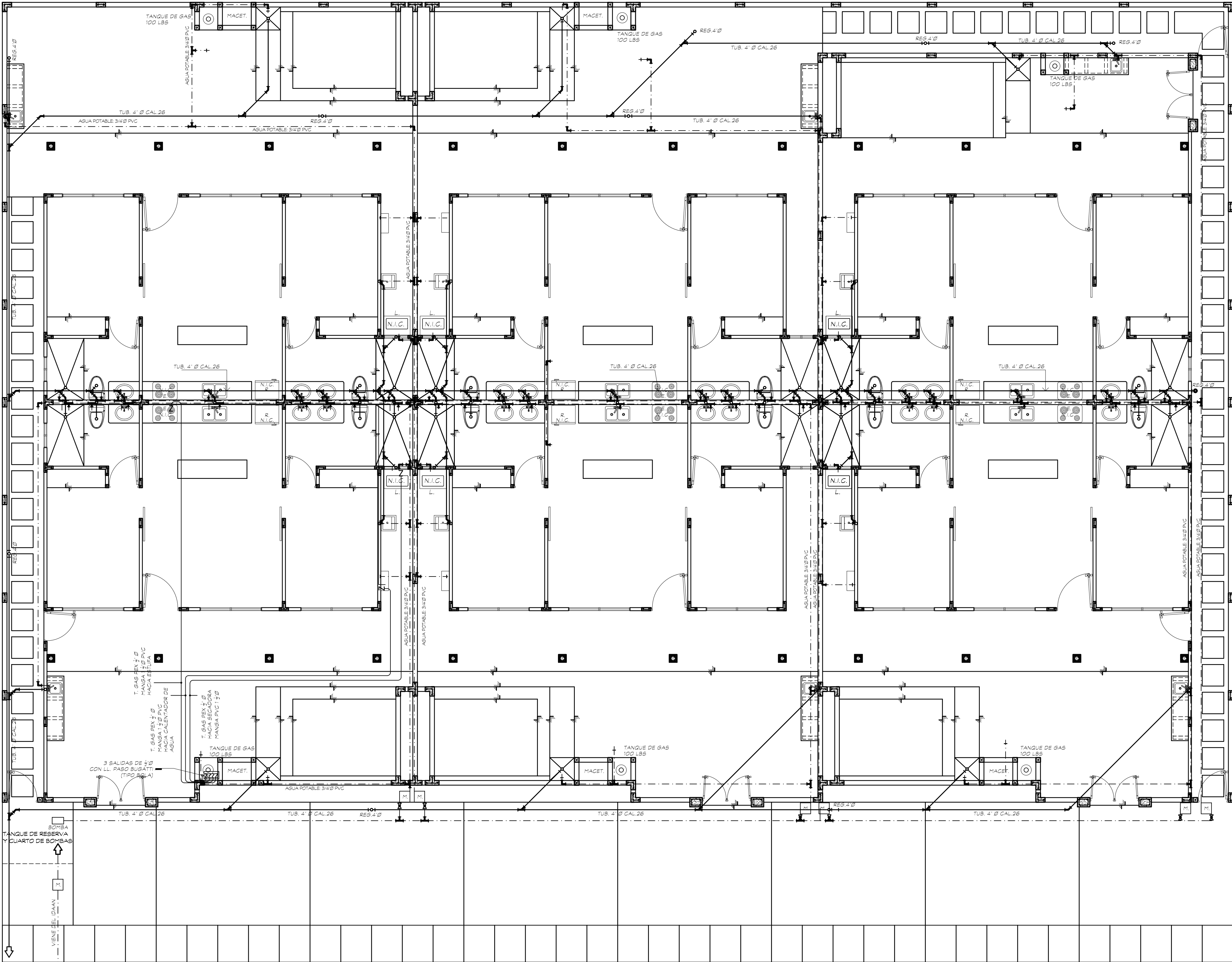
PLANTA DE PLOMERIA: ESC: 1:75 (GENERAL)
