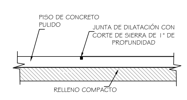
DETALLE ESC. 1:20
