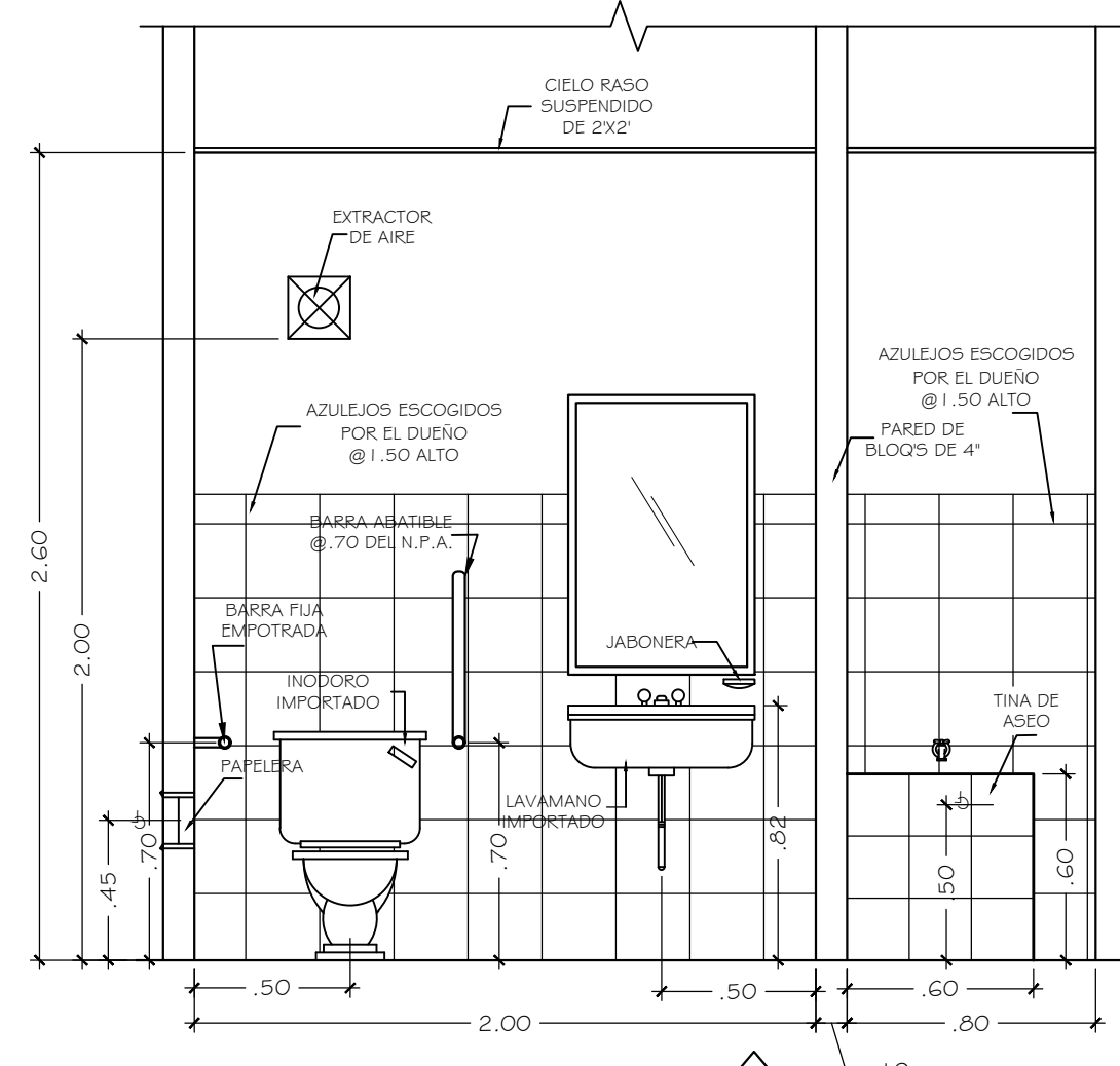
ELEVACION ESC. 1:20
