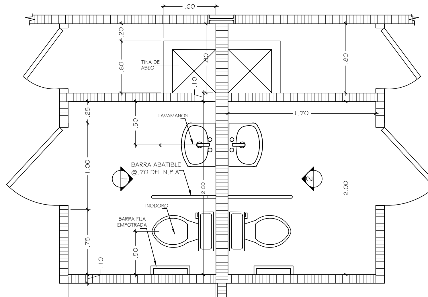
AMPLIACION DE SERV. SANITARIO (LOCALES COMERCIALES) ESC. 1:20
