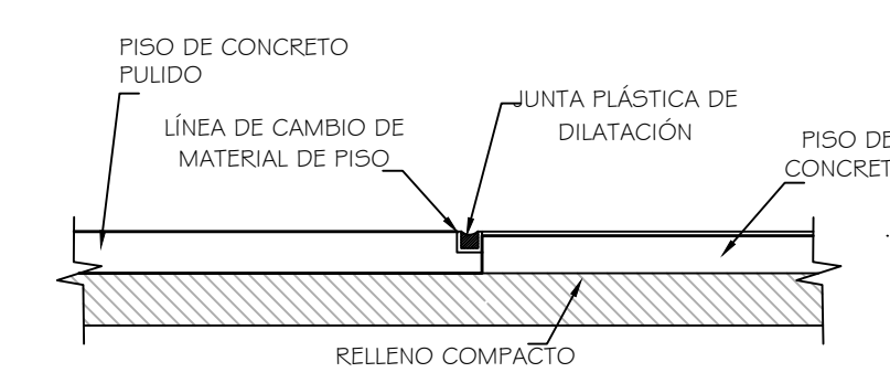
DETALLE ESC. 1:20
