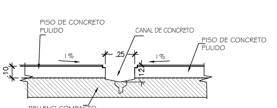
DETALLE ESC. 1:20
