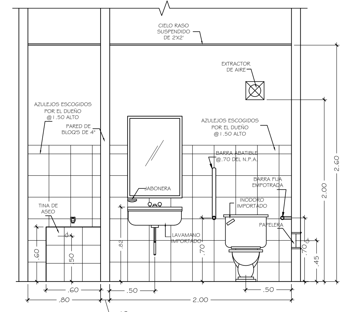
ELEVACION ESC. 1:20
