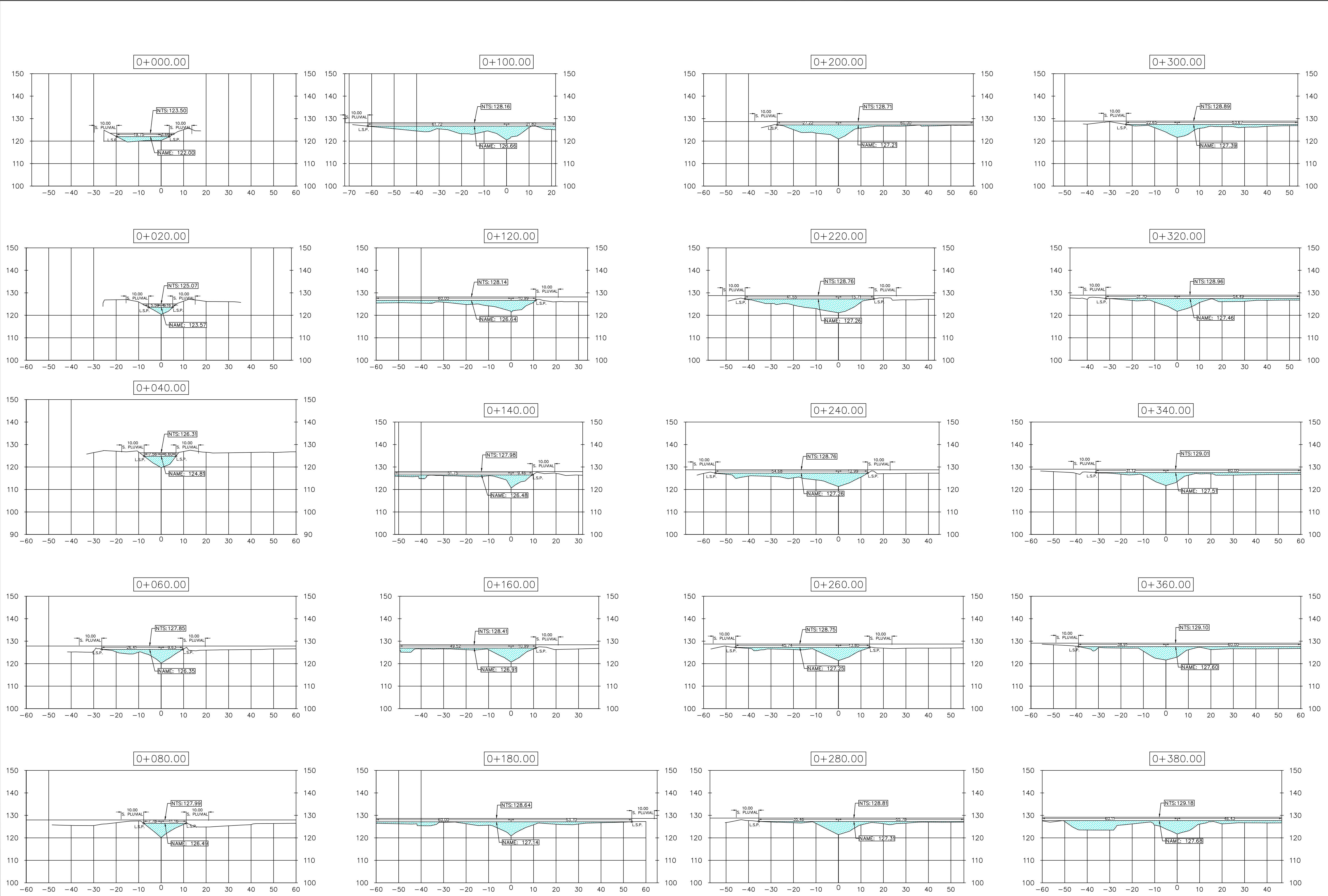
SECCIONES TRANSVERSALES ESCALA: 1:750
