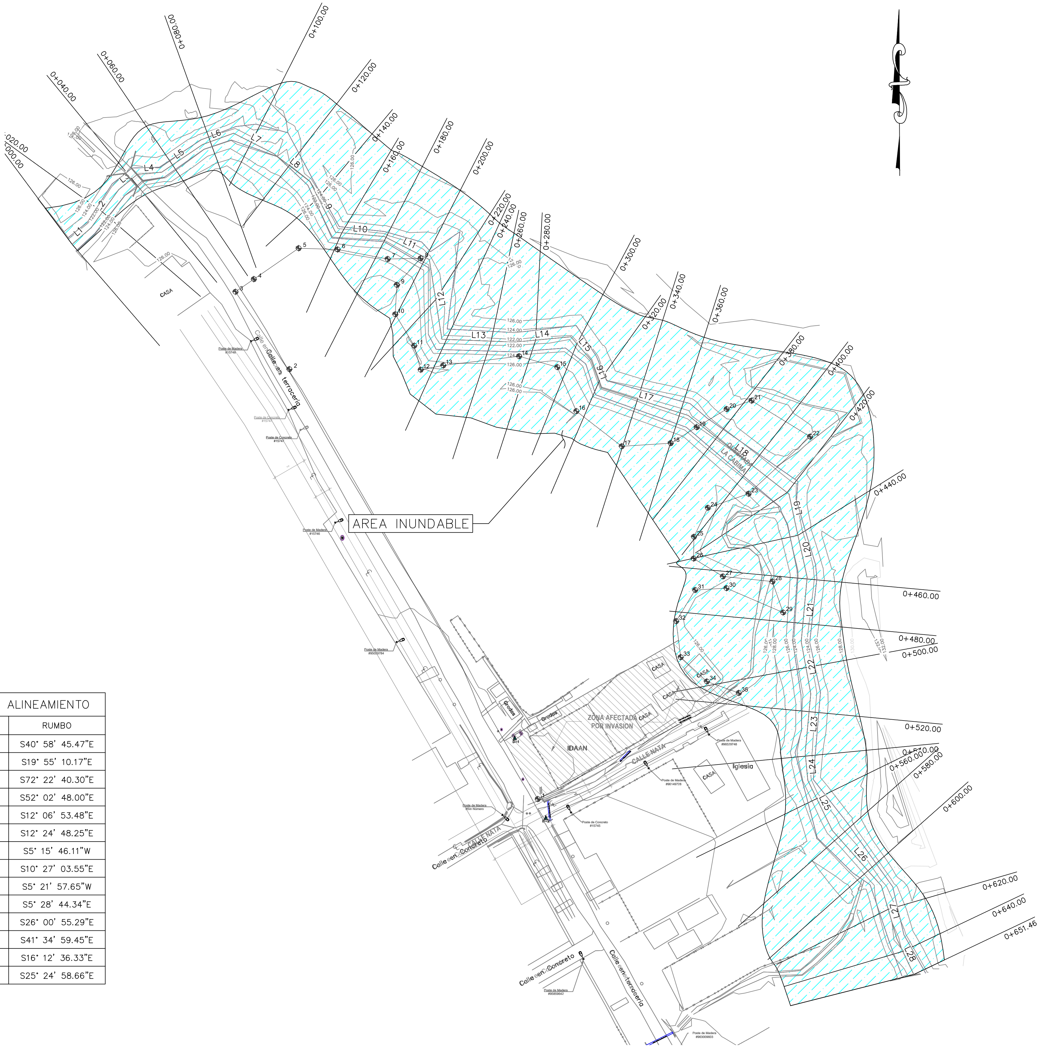
PLANTA GENERAL DEL POLIGONO DE ESTUDIO ESCALA 1:1000
