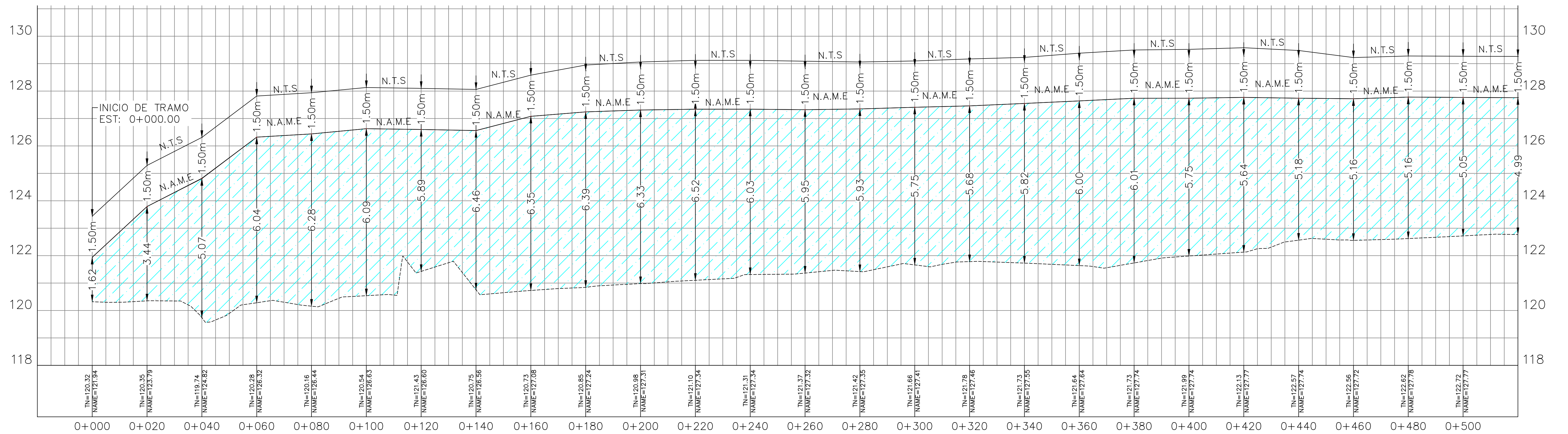
PLANO PERFIL DE QBDA LA CABIMA Q50 - EST. 0K+000 A 0K+520.00 ESCALA 1:750
