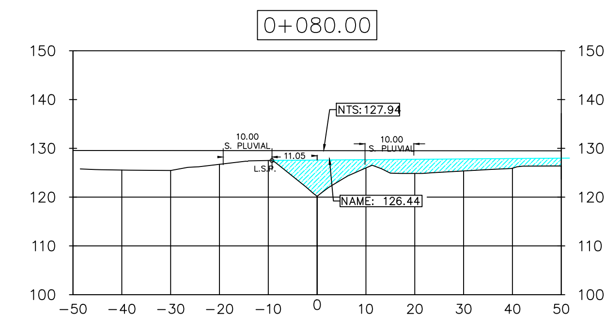
SECCIONES TRANSVERSALES Q50 ESCALA: 1:750
