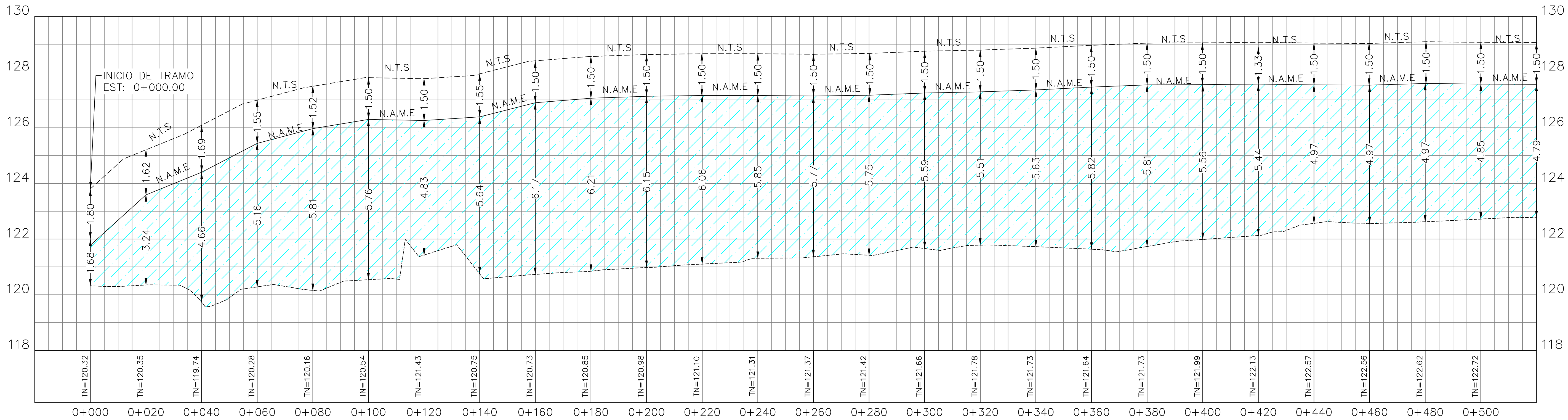
PLANO PERFIL DE QBDA LA CABIMA PARA Q20 - EST. 0K+000 A 0K+520.00 ESCALA 1:750
