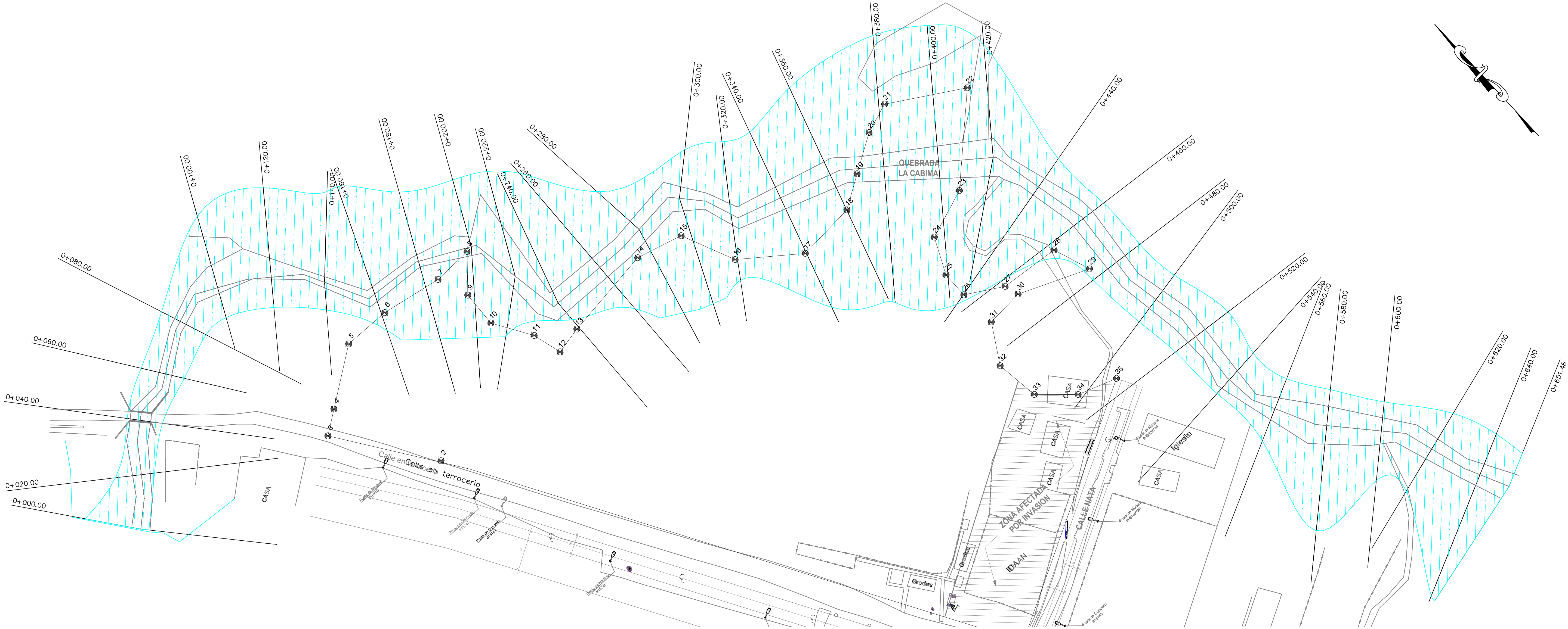
PLANO PERFIL DE QBDA LA CABIMA PARA Q20 - EST. 0K+500 A 0K+641.46 ESCALA 1:750
