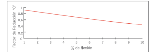
Figura 20. Factor de reducción "C" para el cálculo de la presión crítica de aplastamiento.
