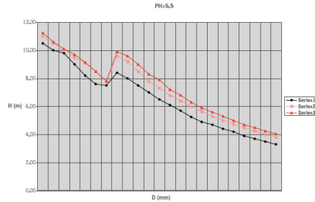
Gráfico 6.1. Rellenos máximos y mínimos, PH=5,5
