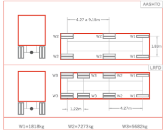
Figura 8. Configuración de ejes y distribución de cargas
