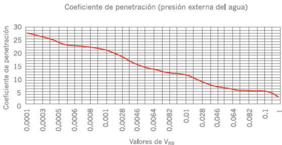
Figura 22. Coeficiente de penetración aD
