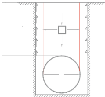
Proporcionalidad de la carga de acuerdo a la Teoría de Marston Figura7: Patrones de carga permanente
