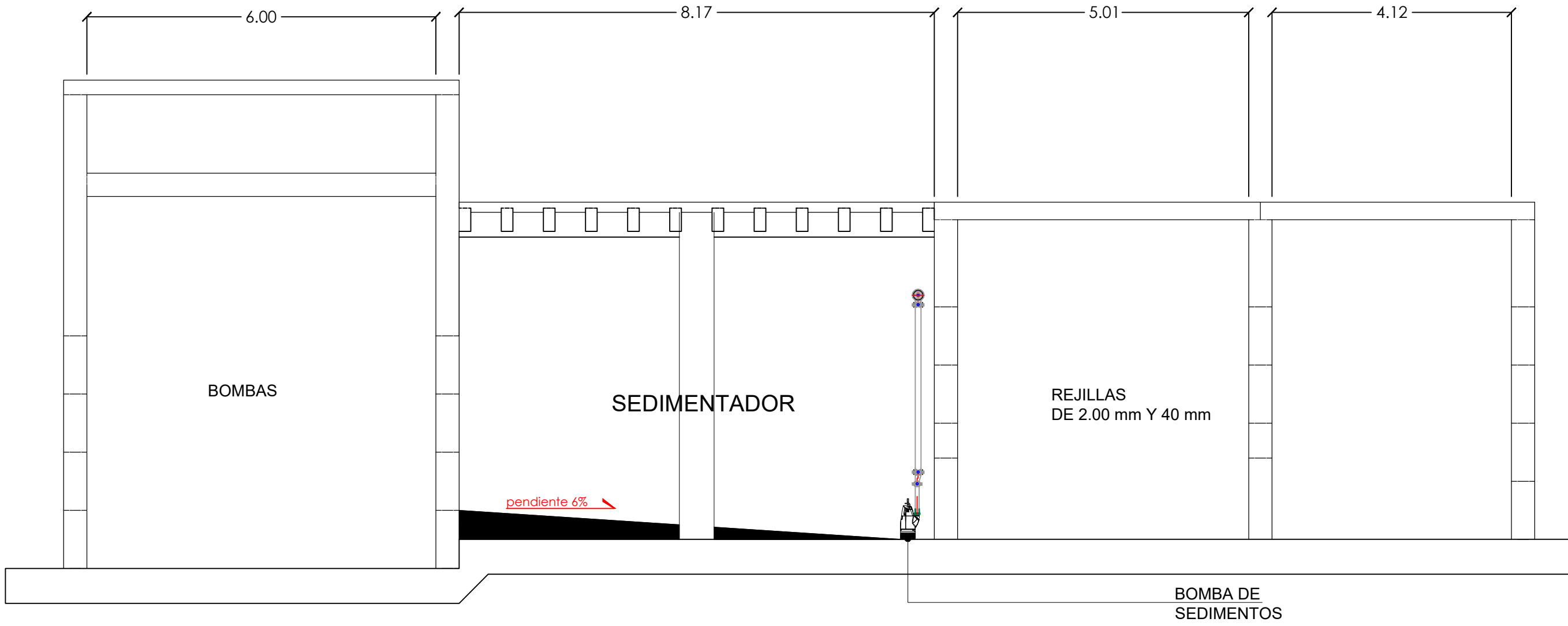
PLANTA ARQUITECTÓNICA EB N°1 ESCALA 1:75
