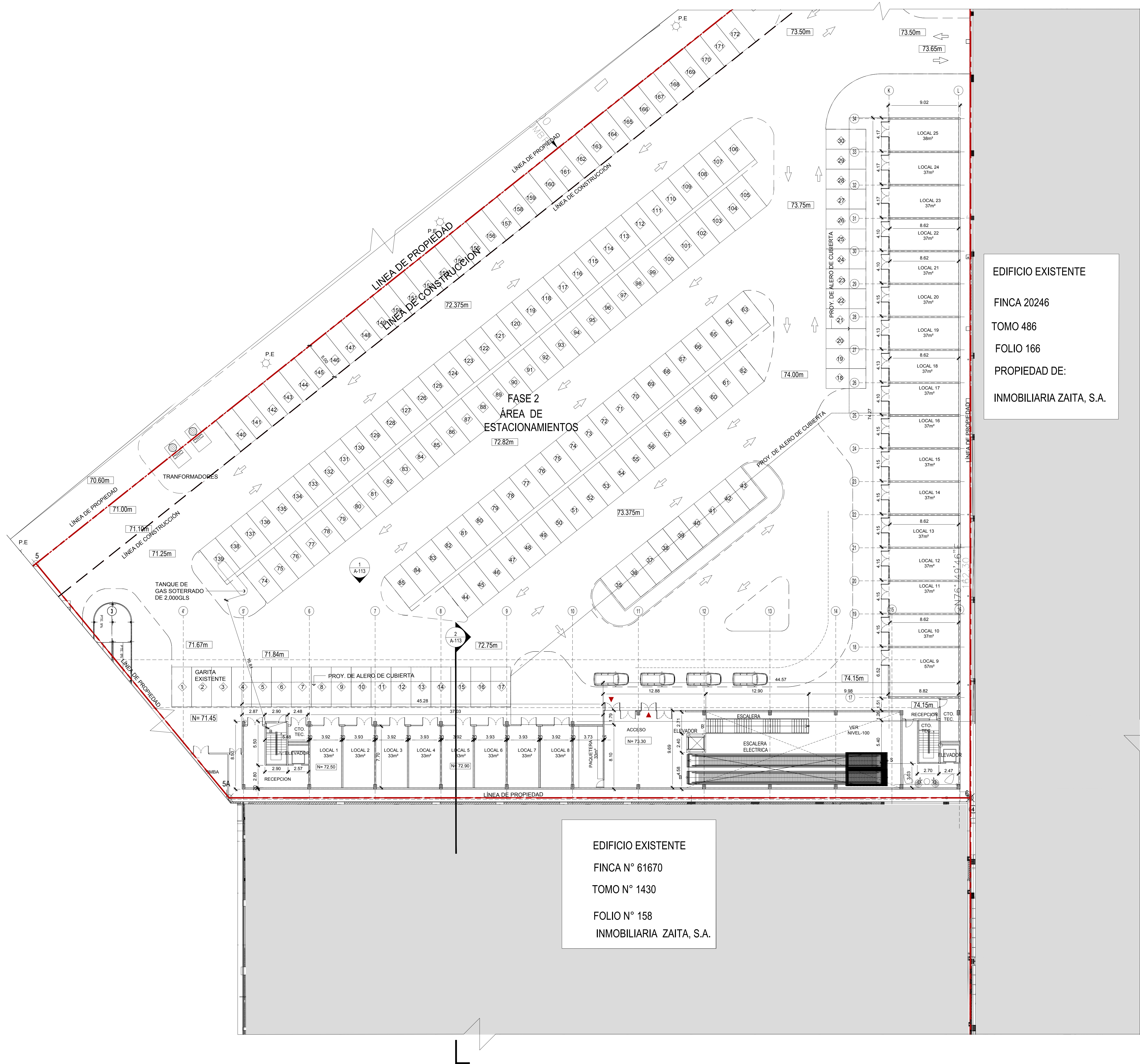
PLANTA ARQUITECTONICA NIVEL 000 FASE 2 (N+74.15) ESCALA 1:200
