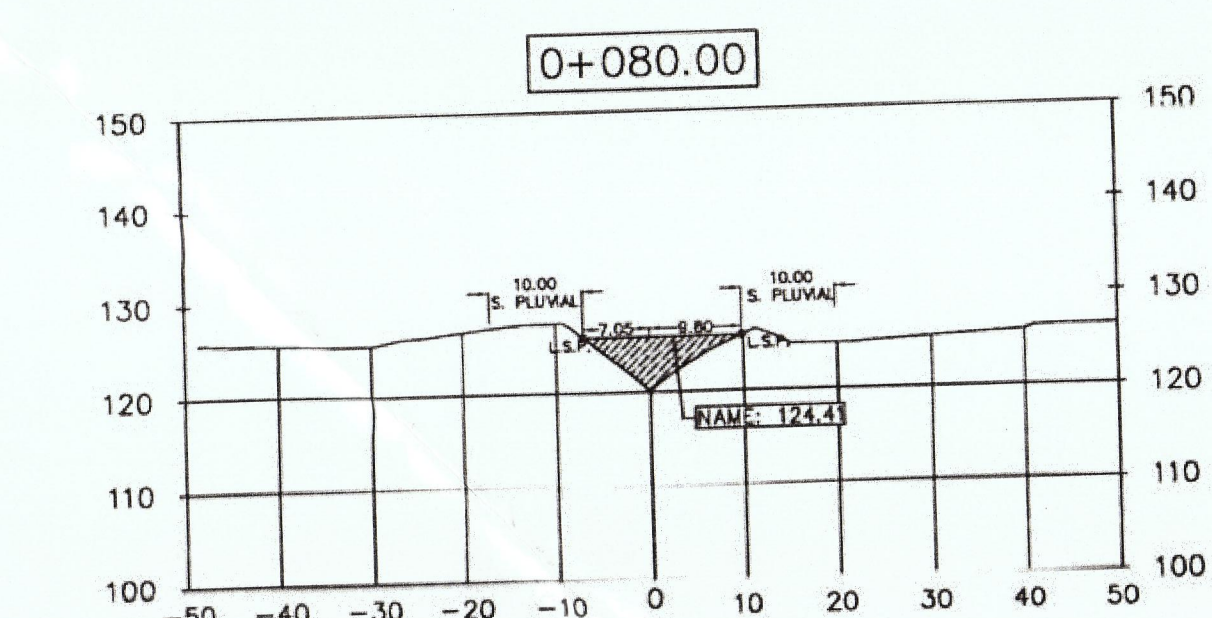
SECCIONES TRANSVERSALES ESCALA: 1:750
