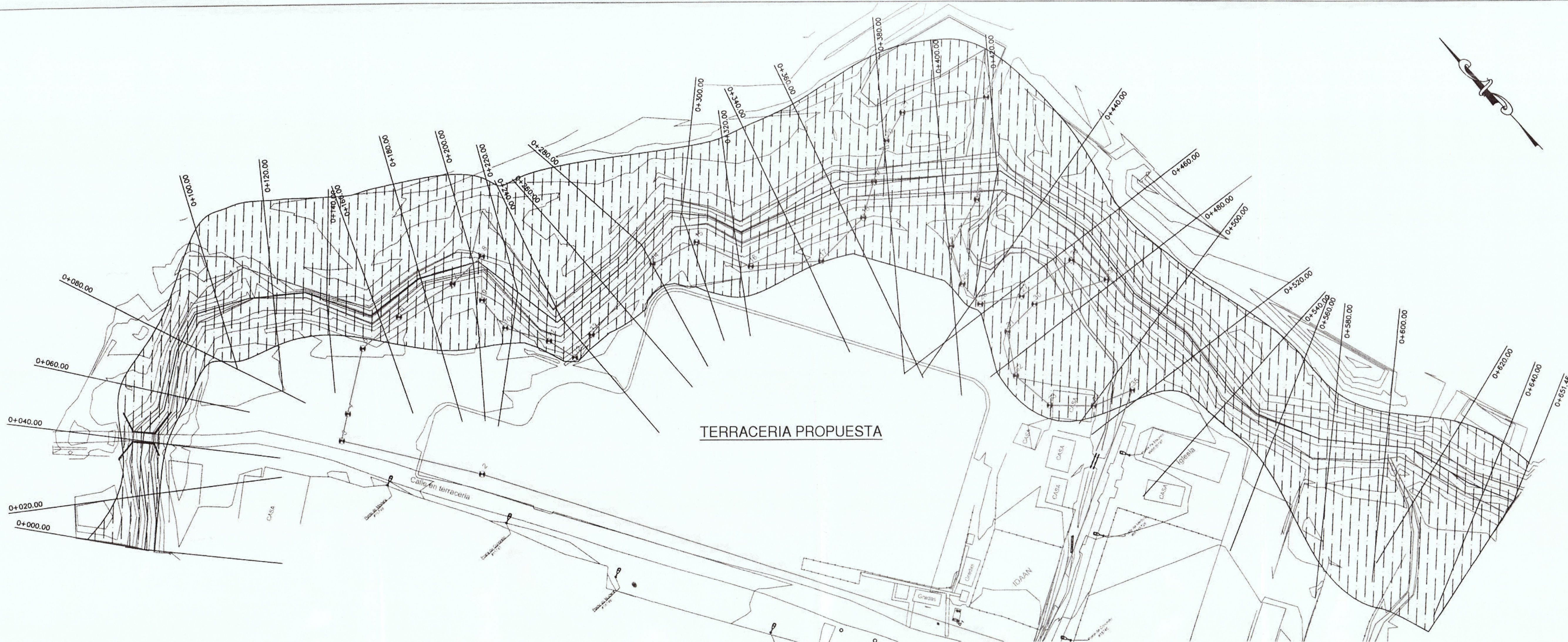
PLANO PERFIL DE QBDA LA CABIMA EST. 0K+500 A 0K+641.46 ESCALA 1:750
