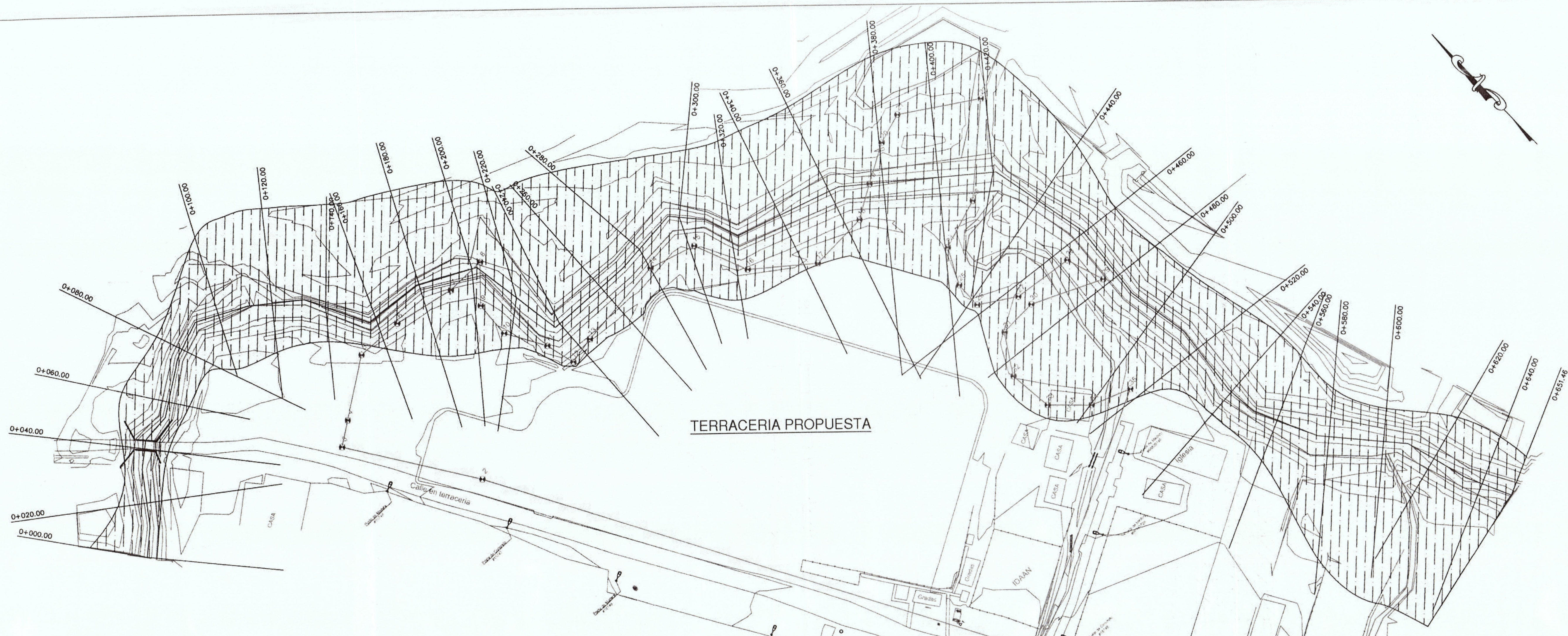
PLANO PERFIL DE QBDA LA CABIMA EST. 0K+000 A 0K+520.00 ESCALA 1:750
